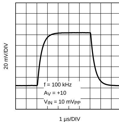
Figure 32. 增益 = 10 时的小信号阶跃响应
