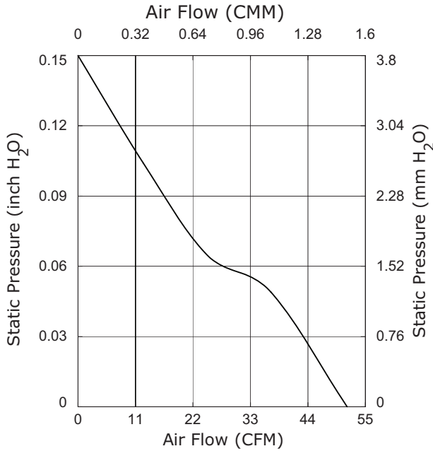
CFM-9225V-130-340
