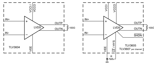
功能方框图
