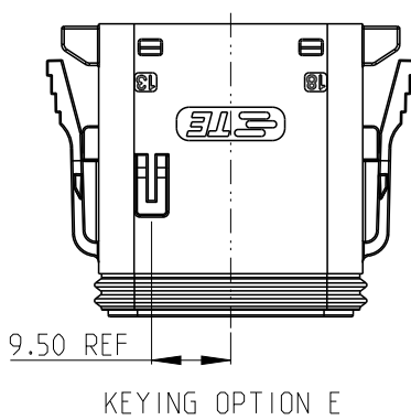
KEYING OPTION E
