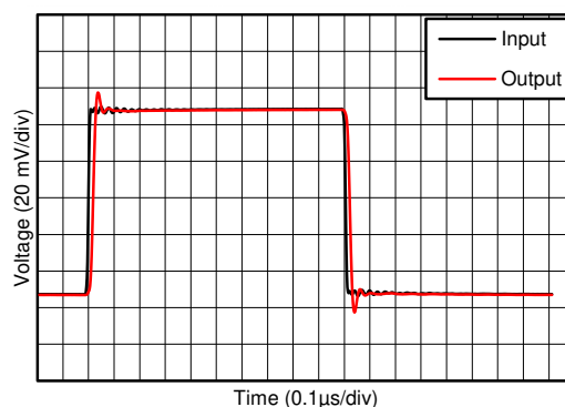
图 7-26. 小信号阶跃响应
