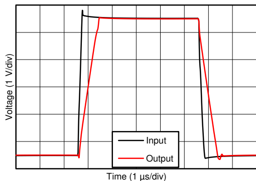
图 7-25. 过载恢复
