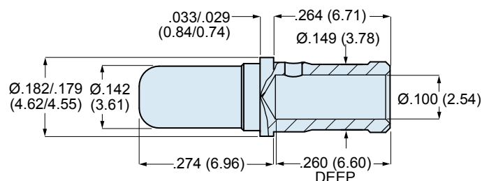
Pin Contact 850-056-0812
