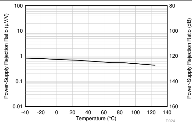
图 6-19. PSRR vs Temperature
