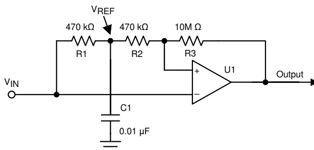
图 8-18. 使用 TLV903x 的脉冲切片器
