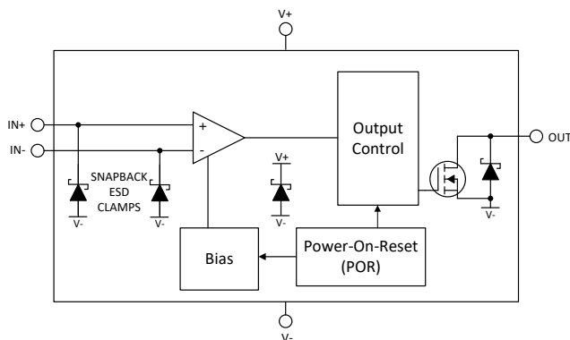
TLV902x 方框图
