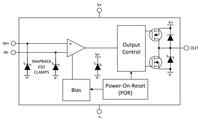
TLV903x 方框图
