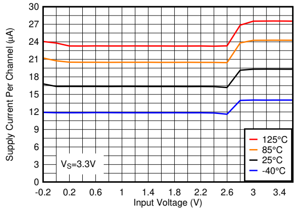
图 6-4. 电源电流与输入电压间的关系, 3.3V
