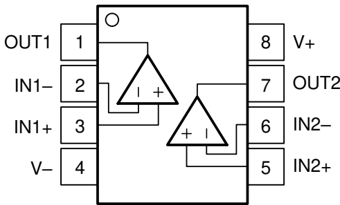
图 5-3. D、DGK、PW、DDF 封装 8 引脚 SOIC、VSSOP、TSSOP、SOT-23-8 顶视图
