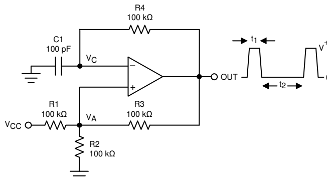
图 8-9. 方波振荡器
