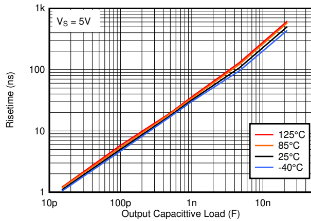
图 6-15. 上升时间与容性负载间的关系
