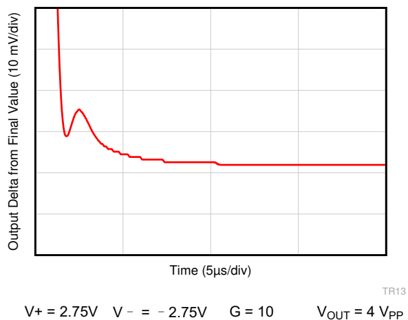
图 7-43. 大信号稳定时间 (上升沿)
