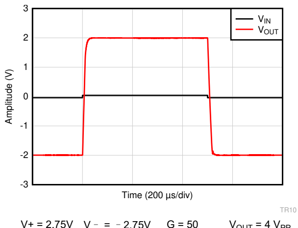
图 7-44. 大信号阶跃响应
