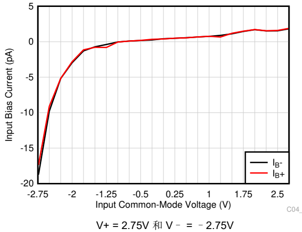
图 7-21. 输入偏置电流与输入共模电压间的关系
