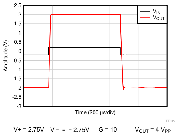
图 7-41. 大信号阶跃响应
