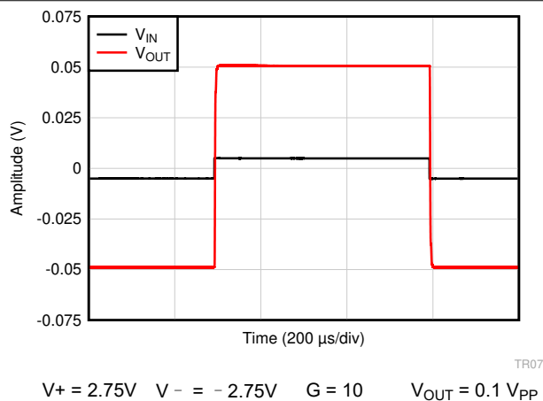
图 7-45. 小信号阶跃响应
