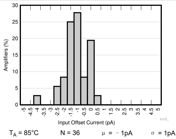
图 7-6. 输入失调电流的典型分布
