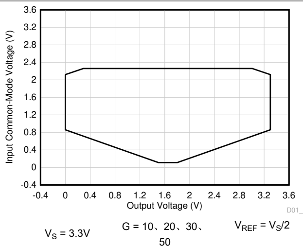
图 7-52. 输入共模电压与输出电压间的关系 (高 CMRR 区域)
