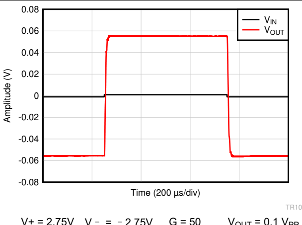
图 7-46. 小信号阶跃响应
