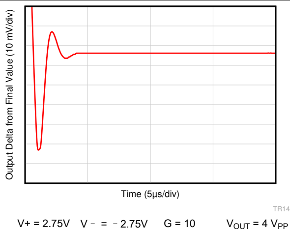
图 7-42. 大信号稳定时间 (下降沿)
