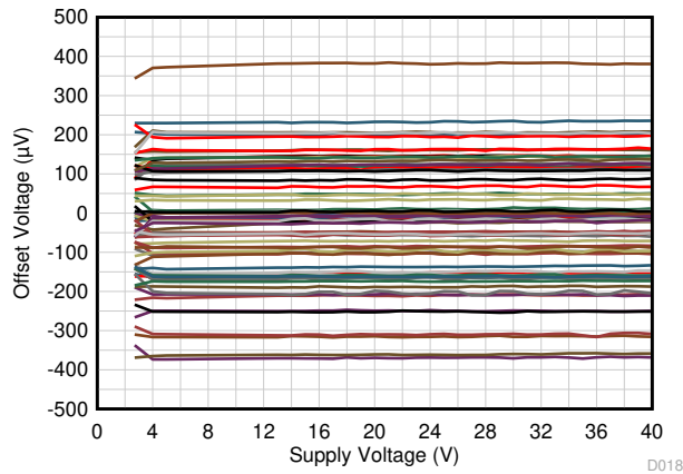
图 5-11. 失调电压与电源间的关系
