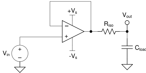
图 6-7. 使用 TLV9351-Q1 扩展容性负载驱动
