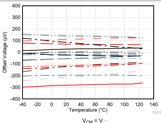
图 5-4. 失调电压与温度间的关系
