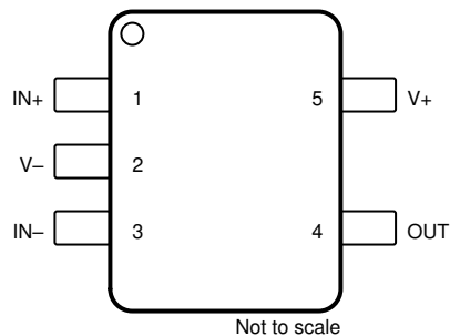
图 4-2. TLV9351-Q1 DCK 封装， 5 引脚 SC70 (顶视图)
