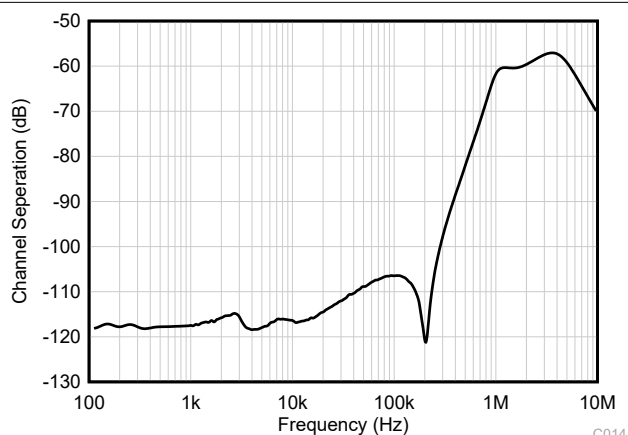
图 5-40. 通道隔离与频率间的关系
