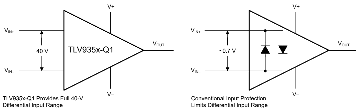
图 6-1. TLV935x-Q1 输入保护不限制差分输入能力
