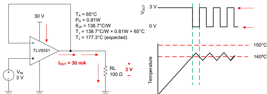
图 6-4. 过热保护
