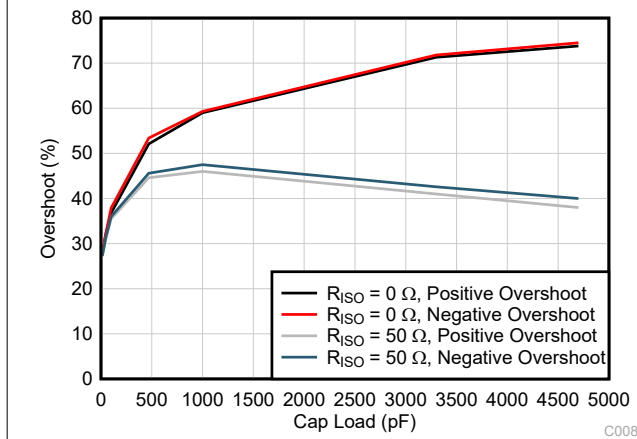
图 6-5. 小信号过冲与容性负载间的关系 ( 100mV 输出阶跃, G = 1 )
