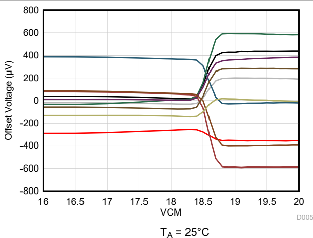
图 5-6. 失调电压与共模电压间的关系 (切换区域)
