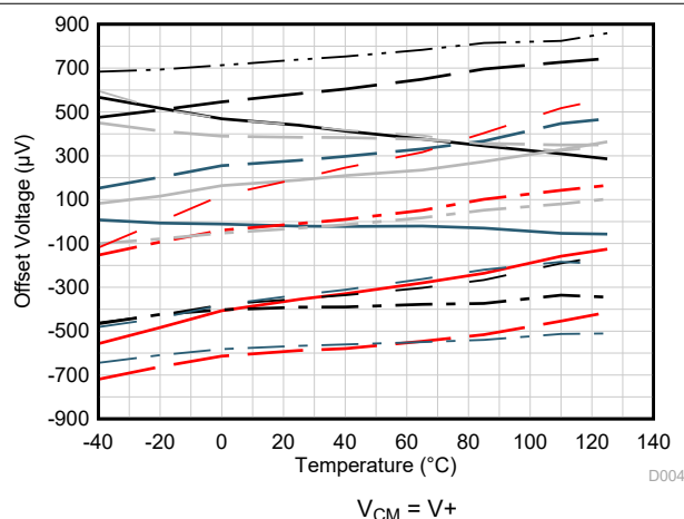
图 5-3. 失调电压与温度之间的关系
