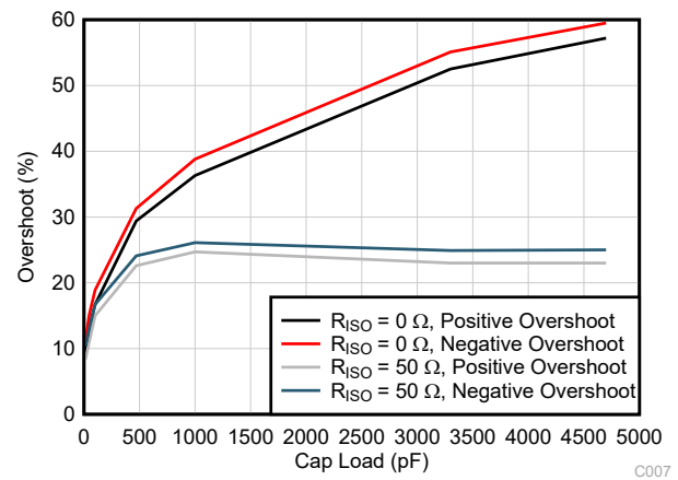
图 6-6. 小信号过冲与容性负载间的关系 ( 100mV 输出阶跃, G = -1 )
