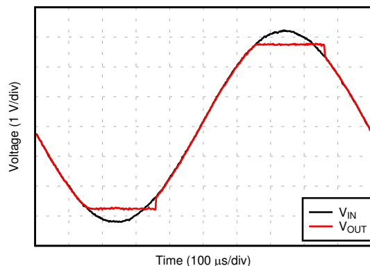
图 6-31. 无相位反转
