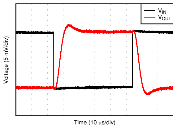
图 6-33. 负过载恢复
