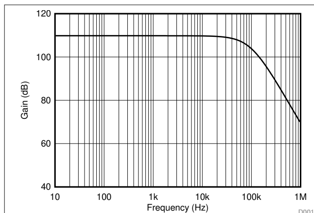
图 9-4. 光电二极管放大器电路交流增益结果
