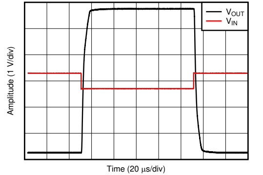
图 7-28. 过载恢复
