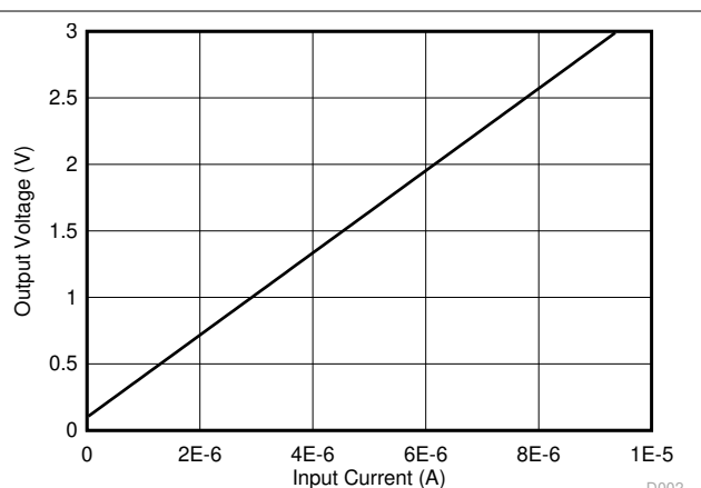
图 9-5. 光电二极管放大器电路直流结果
