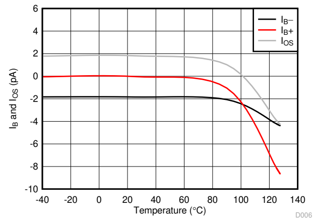
图 7-6. I_B 和 I_{OS} 与温度间的关系
