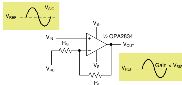
图 45. Noninverting Amplifier
