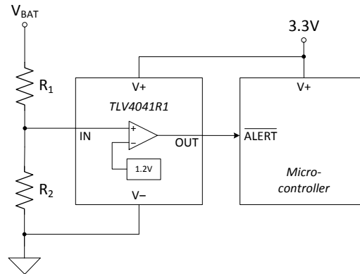
图 9-4. Under-Voltage Detection
