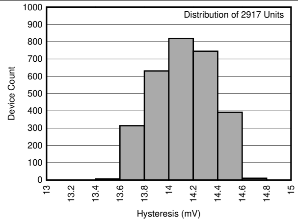
图 34. Hysteresis Histogram
