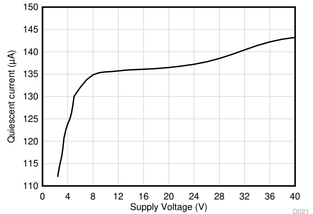
图 6-22. 静态电流与电源电压间的关系
