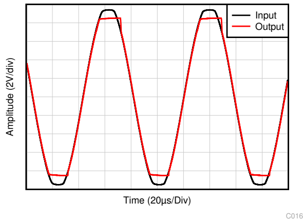
图 6-29. 无相位反转
