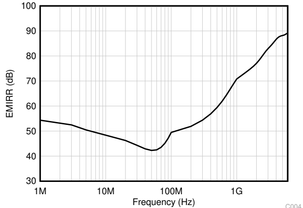
图 6-40. EMIRR (电磁干扰抑制比) 与频率间的关系
