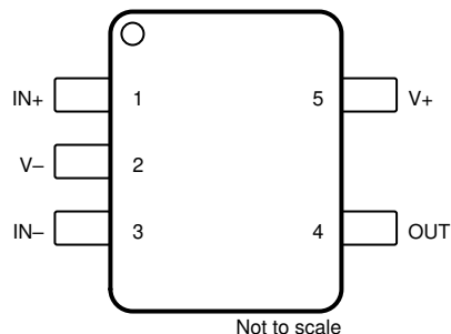
图 5-2. TLV9301 DCK 封装 5 引脚 SC70 顶视图
