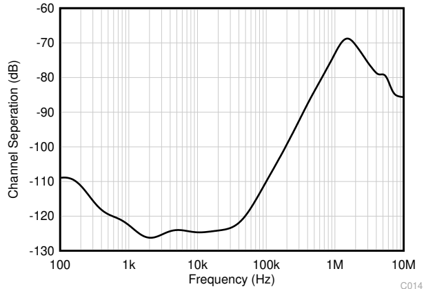
图 6-39. 通道隔离与频率间的关系
