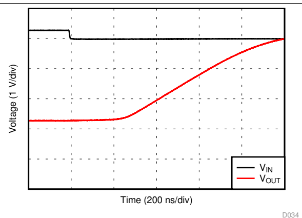
图 22. No Phase Reversal
