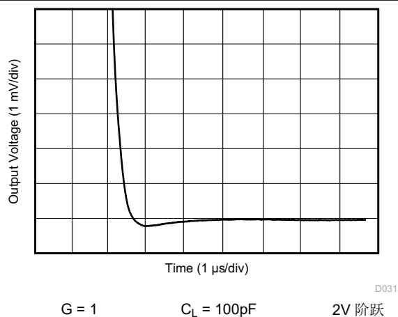
图 6-25. 大信号建立时间 ( 负 )
