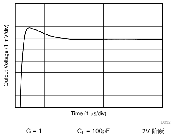
图 6-26. 大信号建立时间 ( 正 )
