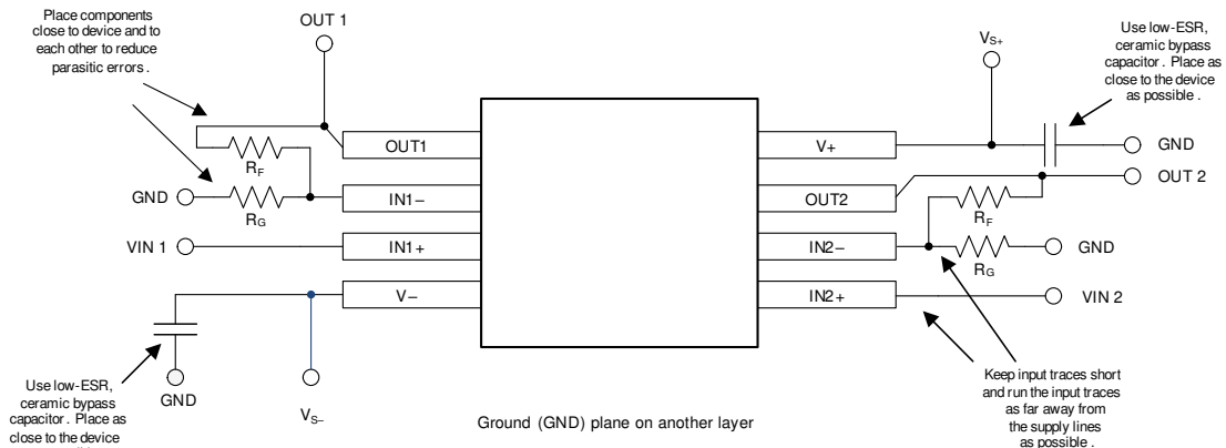
图 10-2. 布局示例
