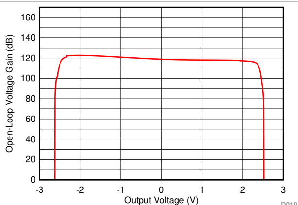
图 6-4. 开环增益与输出电压间的关系
