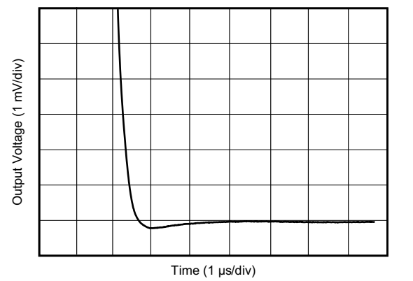
图 6-26. 大信号建立时间 ( 负 )
