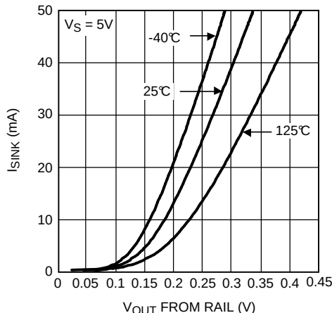
图 16. 灌电流与输出电压间的关系 (LMV652)
