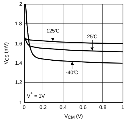
图 6. V_{OS} 与 V_{CM} 间的关系
