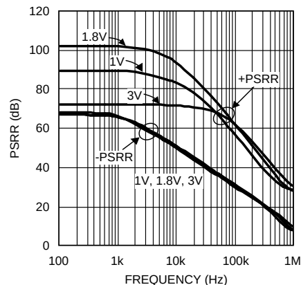
图 40. PSRR 与频率间的关系
