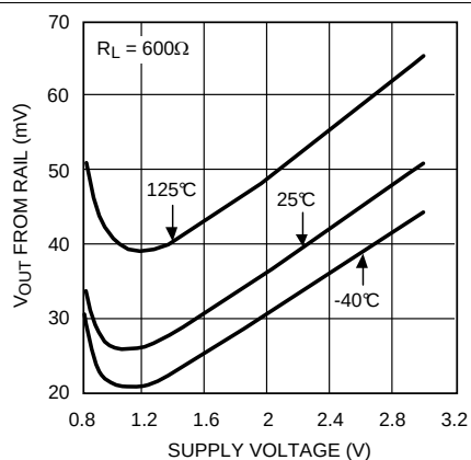
图 23. 正输出摆幅与电源电压间的关系
