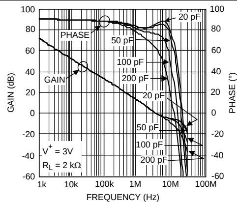
图 29. 开环增益和相位与容性负载
