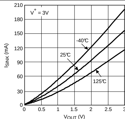
图 20. 灌电流与输出电压间的关系
