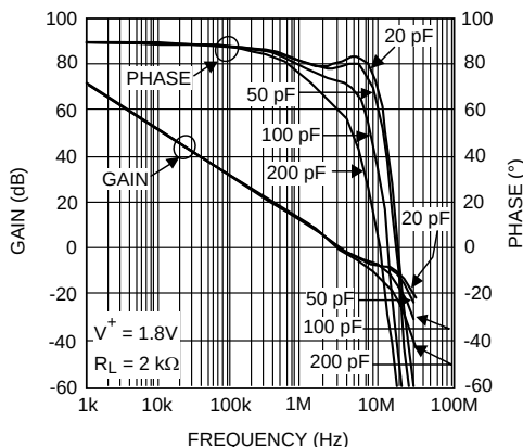
图 27. 开环增益和相位与容性负载
