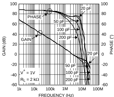
图 25. 开环增益和相位与容性负载
