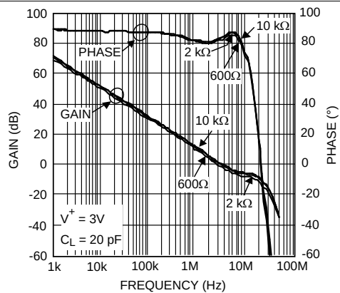
图 30. 开环增益和相位与阻性负载
