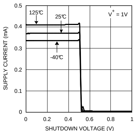
图 3. 电源电流与关断电压间的关系
