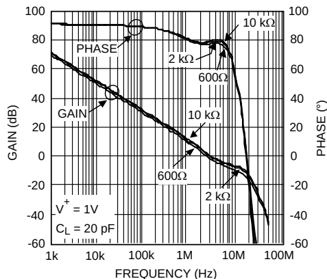
图 26. 开环增益和相位与阻性负载
