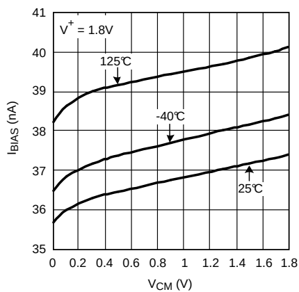
图 11. I_{BIAS} 与 V_{CM} 间的关系
