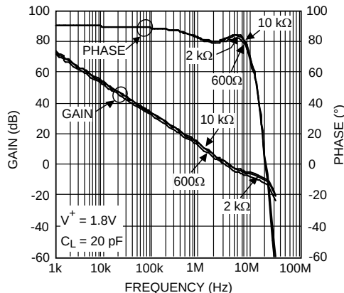
图 28. 开环增益和相位与阻性负载
