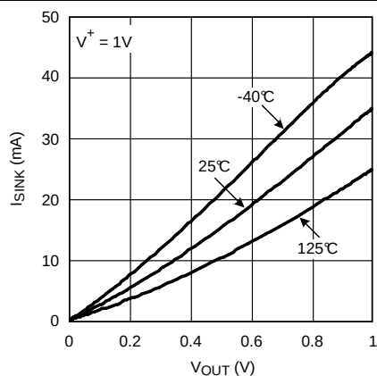
图 16. 灌电流与输出电压间的关系
