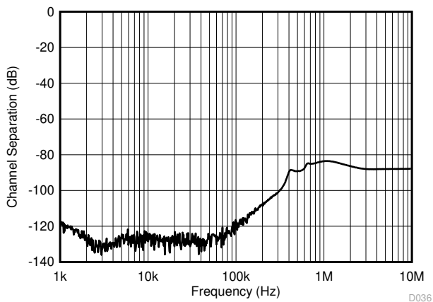
图 7-36. 通道分离
