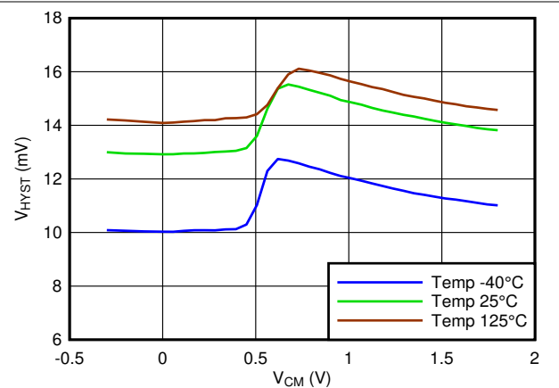
图 6-12. Hysteresis vs V_{CM}
