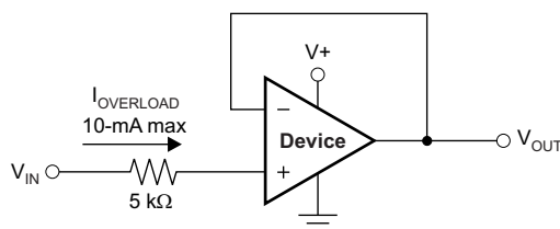
图 20. 输入电流保护
