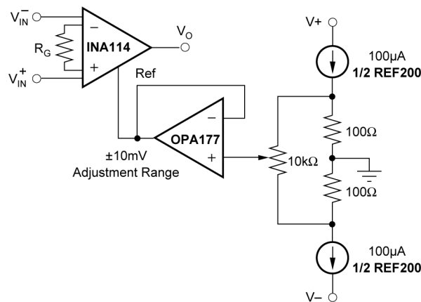
图 6-2. Optional Trimming of Output Offset Voltage.
