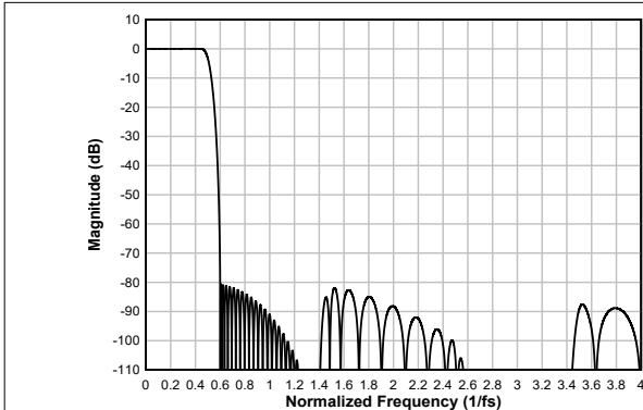
图 8-9. 线性相位抽取滤波器幅度响应
