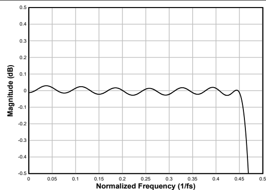
图 8-21. 线性相位内插滤波器通带纹波
