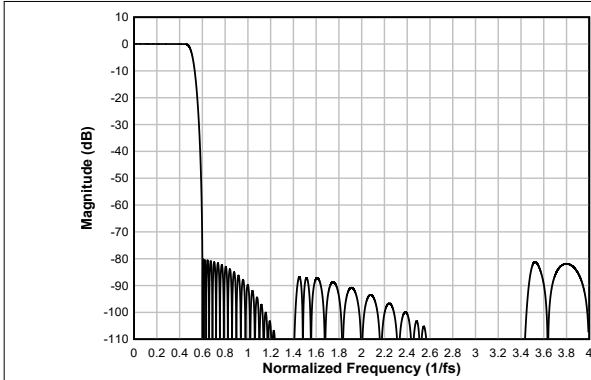
图 8-7. 线性相位抽取滤波器幅度响应
