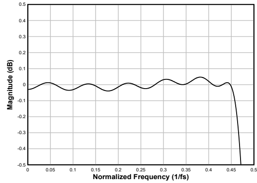
图 8-12. 线性相位抽取滤波器通带纹波
