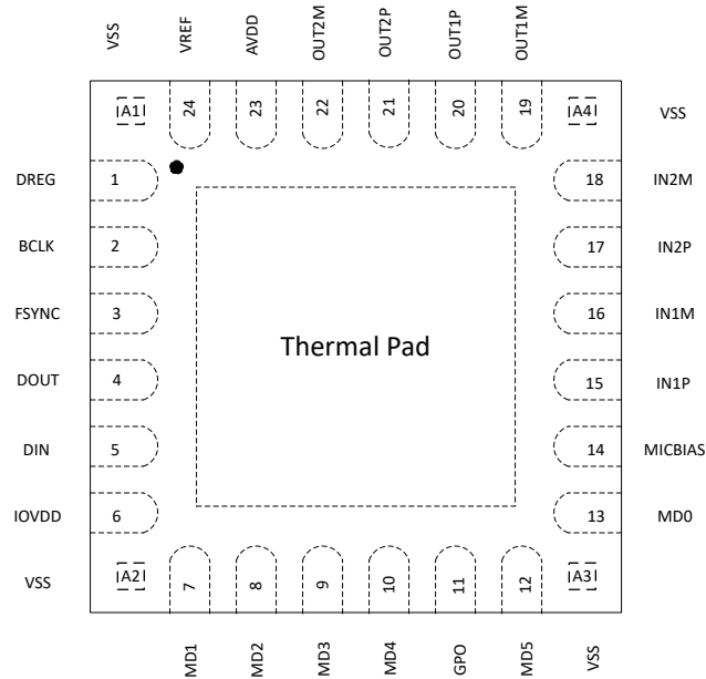
图 5-1. TAC5142 引脚排列
