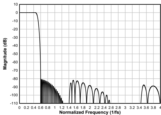
图 7-22. 线性相位抽取滤波器幅度响应
