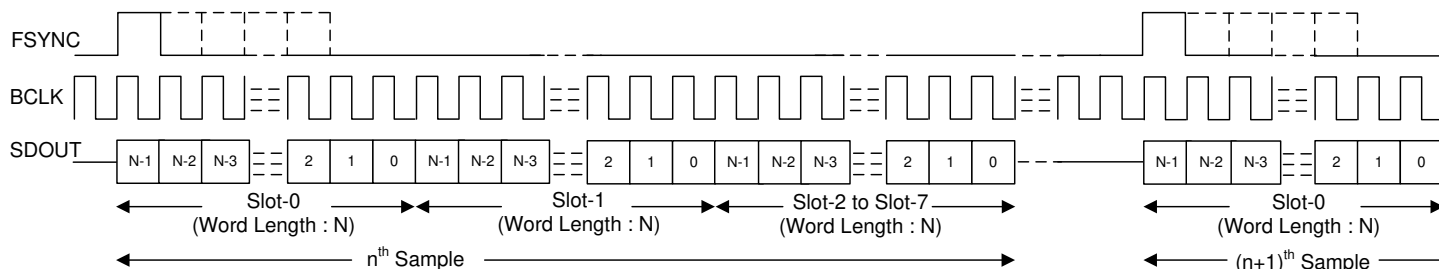
图 7-2. TDM 模式标准协议时序 (PASI TX OFFSET = 0)
