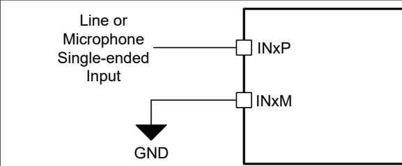
图 7-15. 单端直流耦合输入连接
