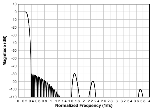
图 7-30. 线性相位抽取滤波器幅度响应
