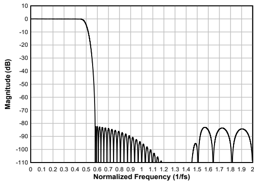
图 7-42. 线性相位内插滤波器幅度响应
