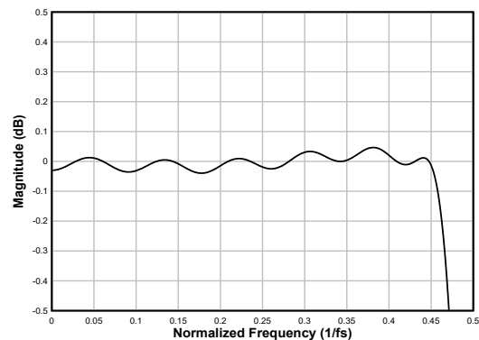
图 7-23. 线性相位抽取滤波器通带纹波
