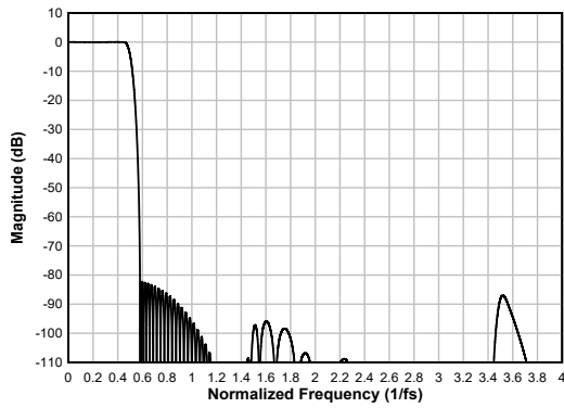
图 7-28. 线性相位抽取滤波器幅度响应
