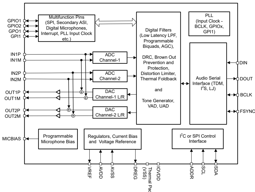
图 7-1. 功能方框图
