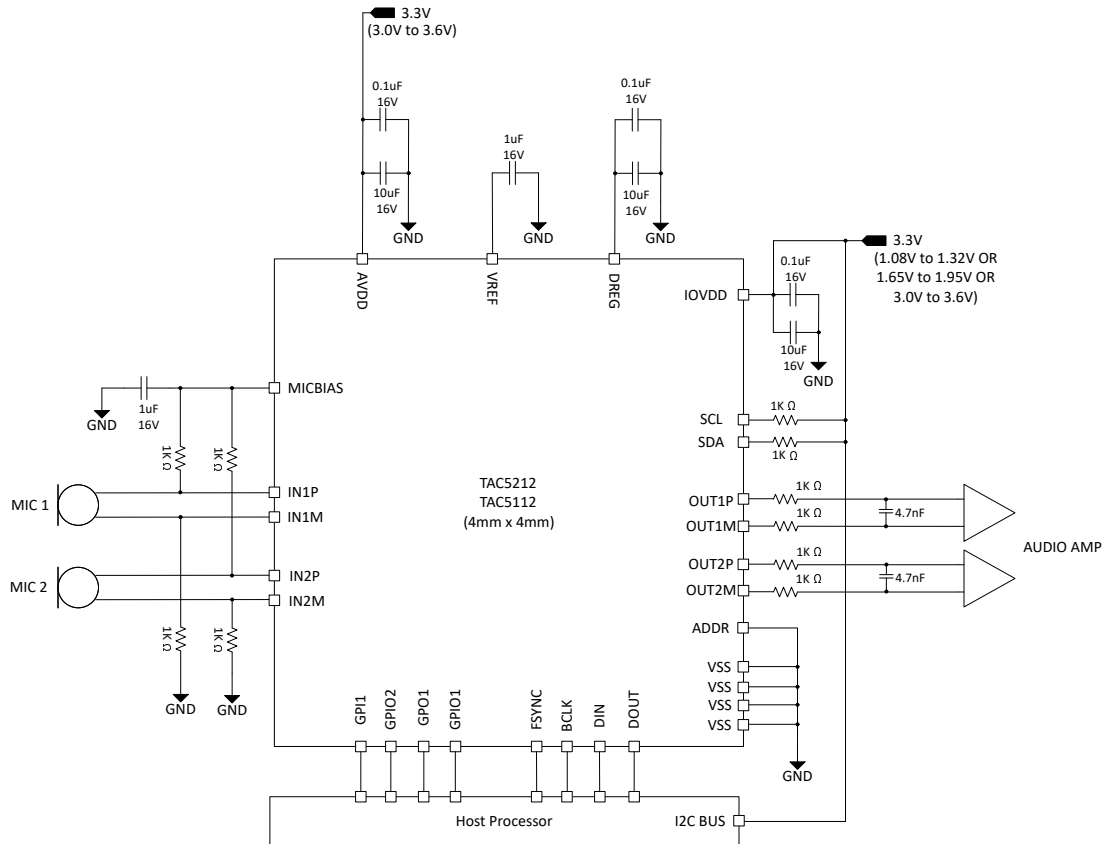
图 8-1. 具有立体声线路输出的立体声麦克风方框图
