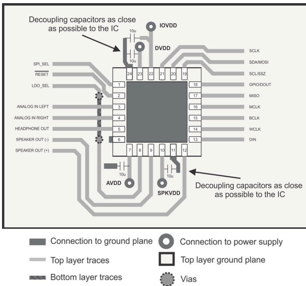
图 9-6. 布局图
