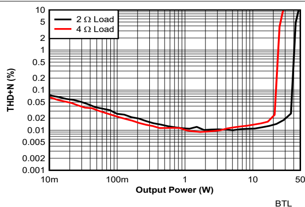
图 7-19. THD+N vs Power - 384 kHz
