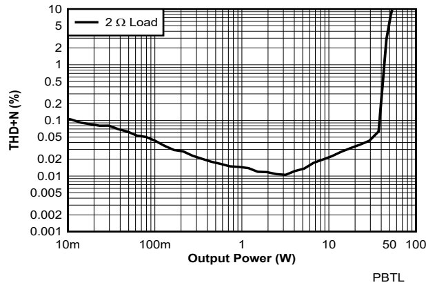
图 7-37. THD+N vs Power - PBTL - 384 kHz
