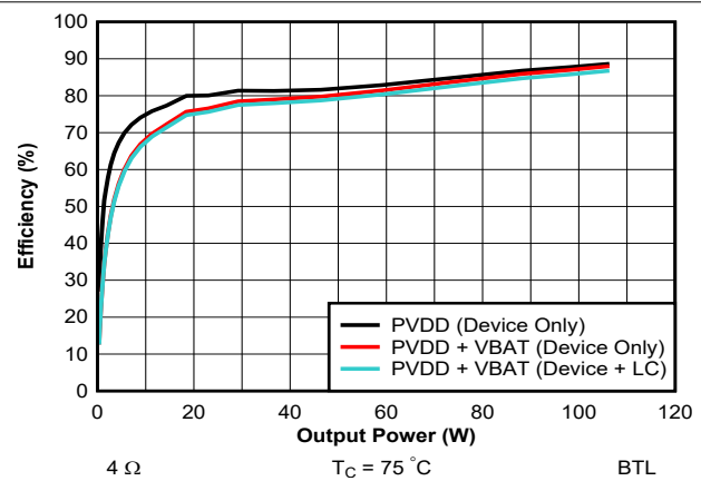
图 7-6. Efficiency vs Output Power - 14.4 V - 4 Ω
