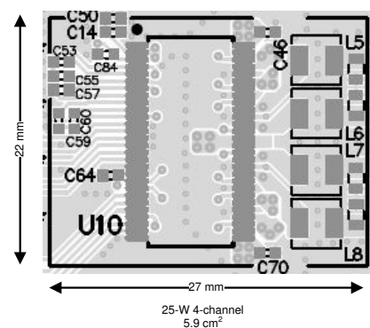
PCB 区域
