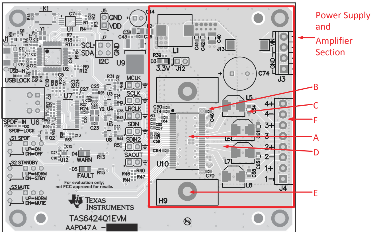
图 10-4. EVM Layout
