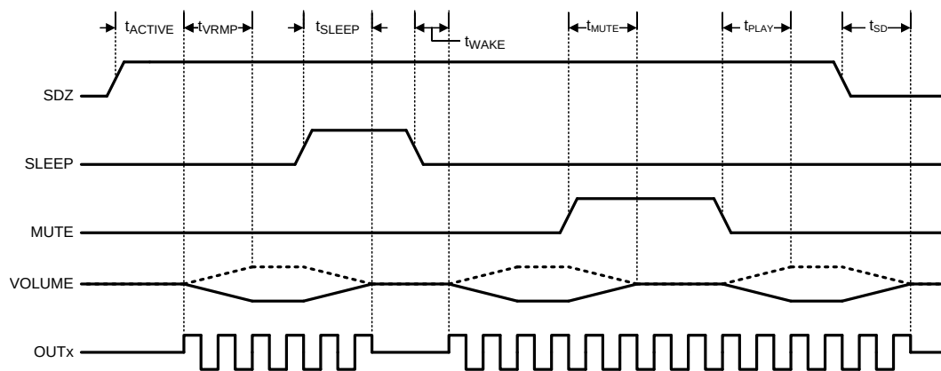
图 4. Mode Timing
