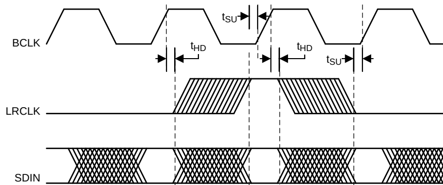
图 1. SAIF Timing
