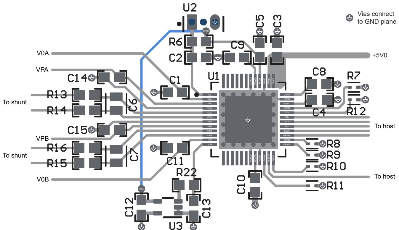
图 10-8. Layout Example
