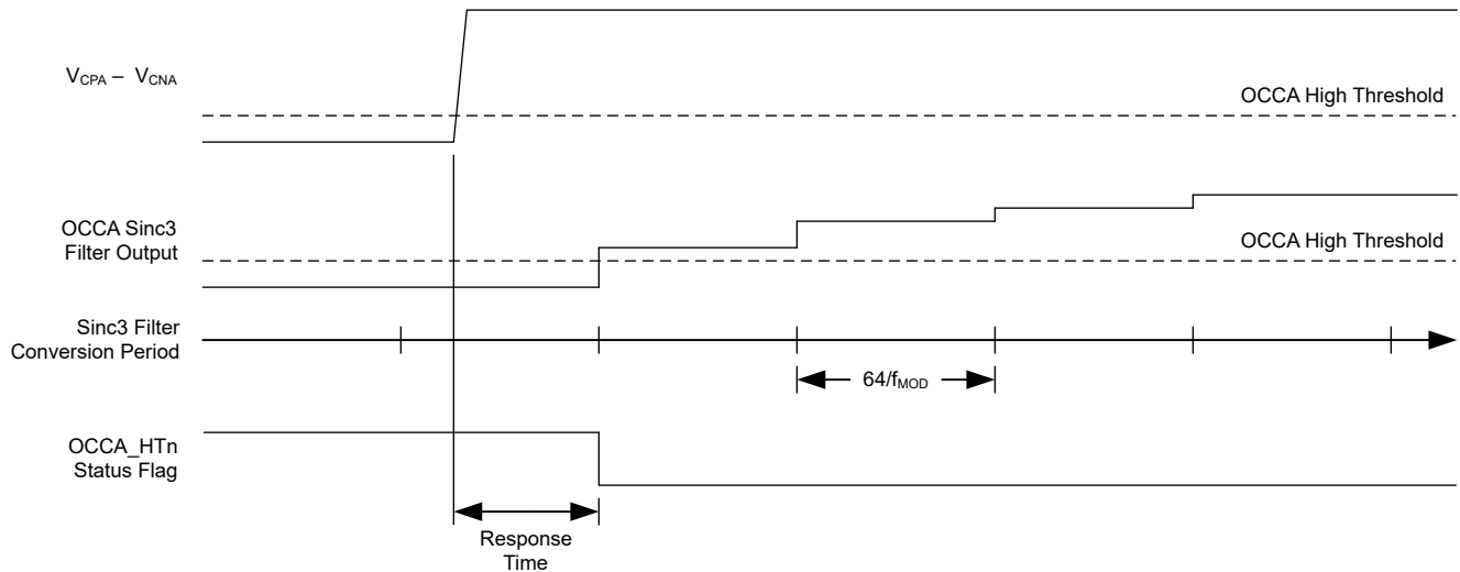
图 9-14. OCCA 行为与大的输入过冲
