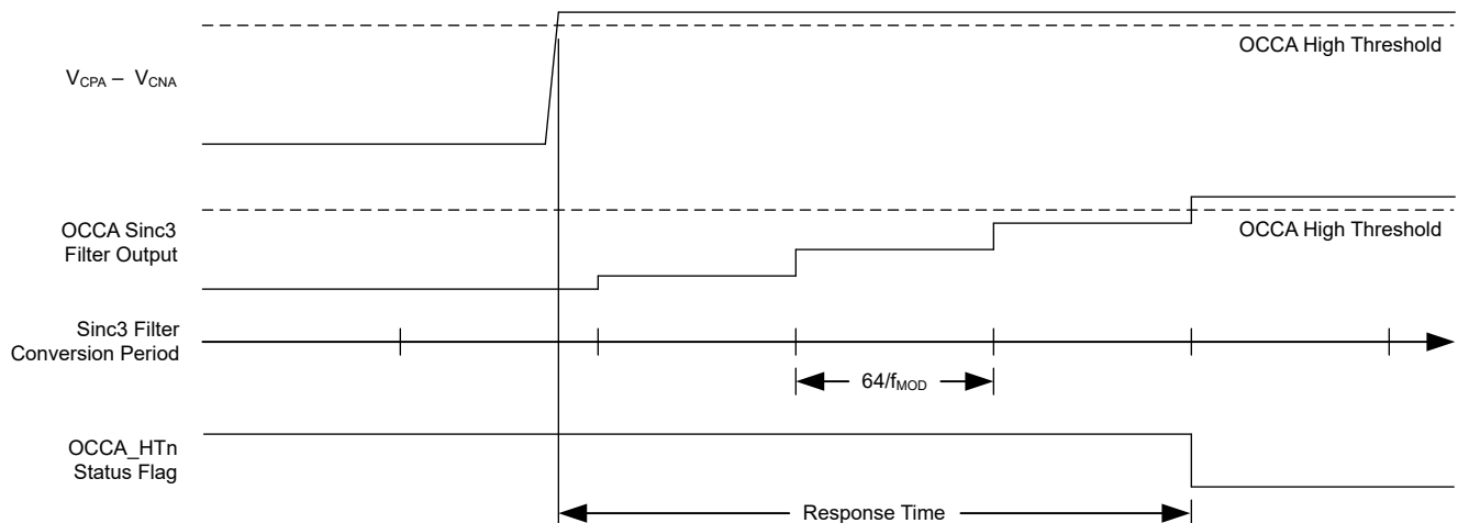
图 9-15. OCCA 行为与小的输入过冲
