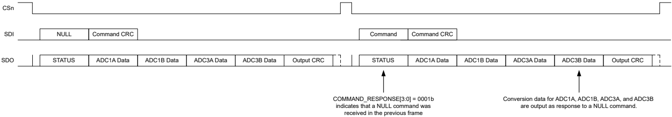
图 9-31. NULL Command Frame
