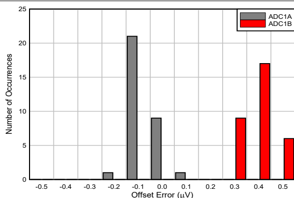
图 7-2. ADC1y Offset Error Histogram
