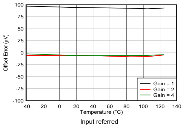
图 7-9. ADC2y Offset Error vs Temperature
