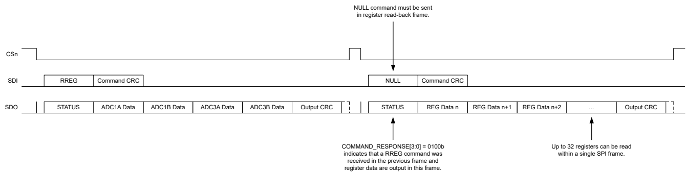
图 9-37. RREG Command Frame
