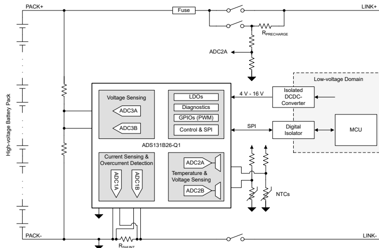
EV BMS 电池包监测系统方框图
