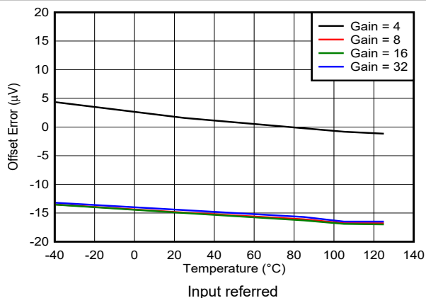
图 7-23. OCCy Offset Error vs Temperature
