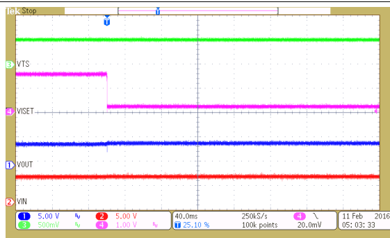
图 17. TS Enable and Disable
