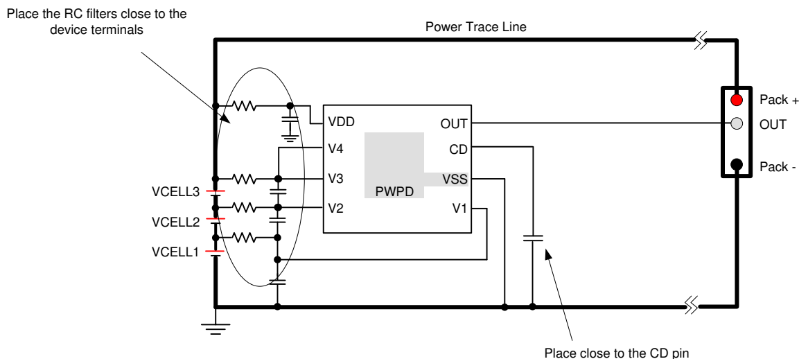
图 11-1. Layout
