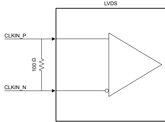
图 8-4. LVDS 输入接口
