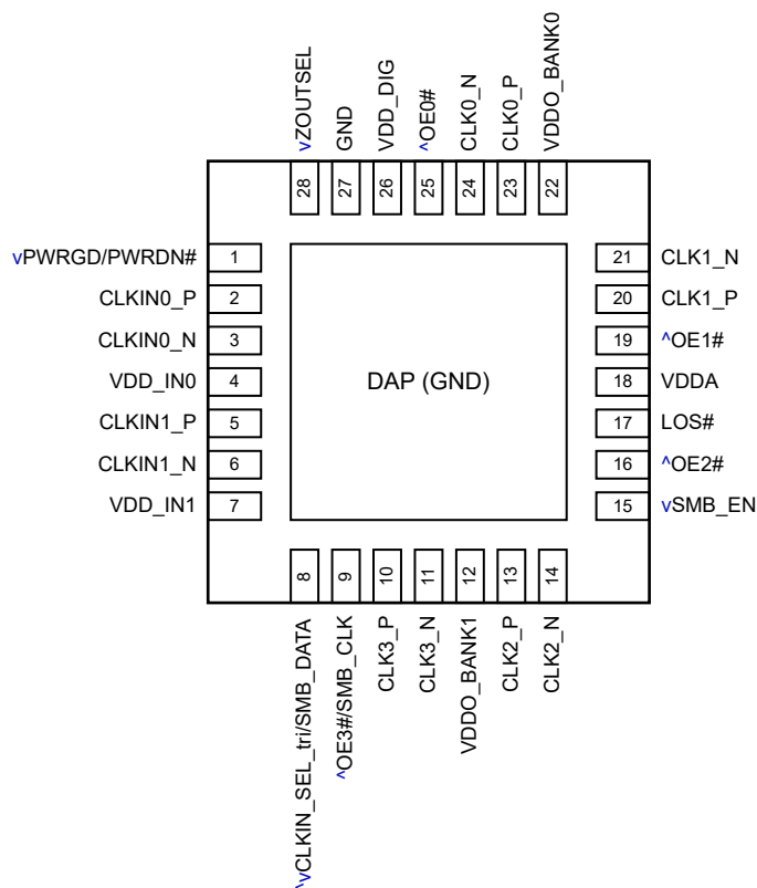
图 5-3. LMKDB1204 4mm x 4mm 28 引脚 QFN
