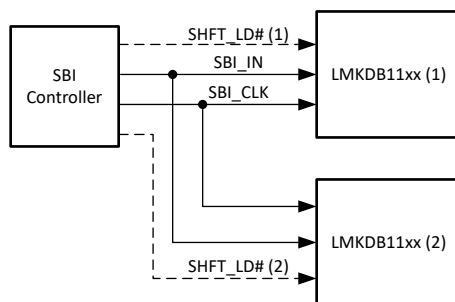
图 8-13. SBI 星型拓扑
