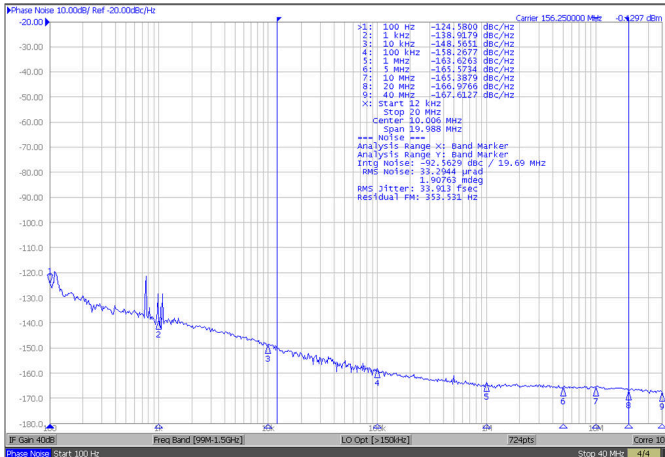
图 10-3. 参考时钟 + LMKDB 相位噪声
