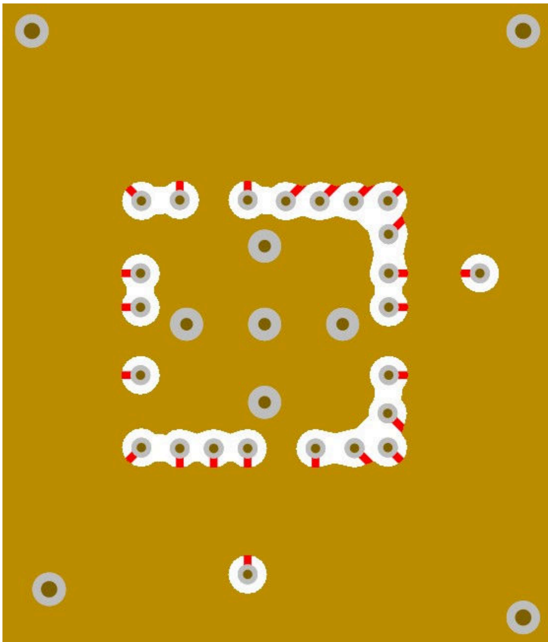
图 10-7. 布局示例 - GND 层
