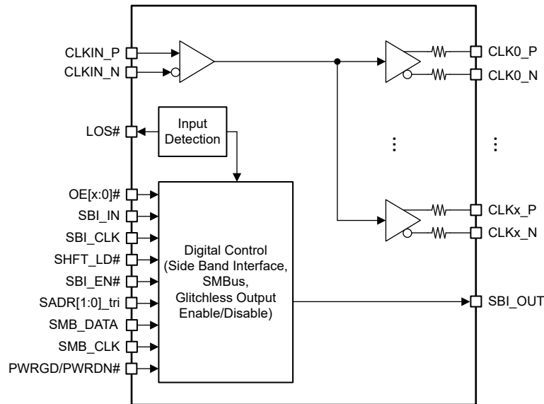
图 8-1. LMKDB1120 或 LMKDB1108 方框图
