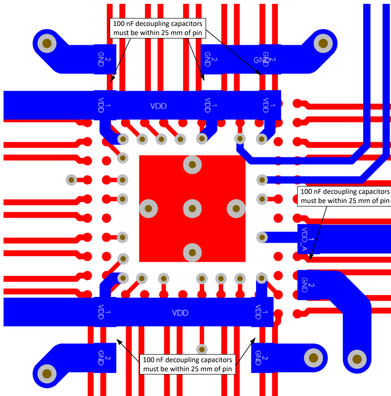
图 10-8. 布局示例 - 底层
