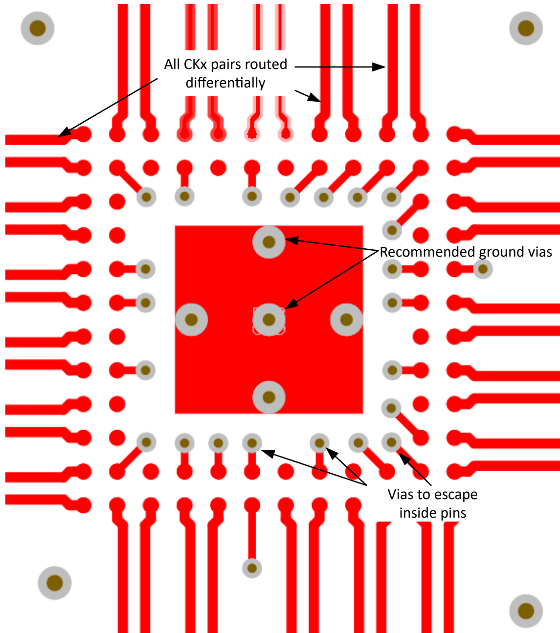
图 10-6. 布局示例 - 顶层
