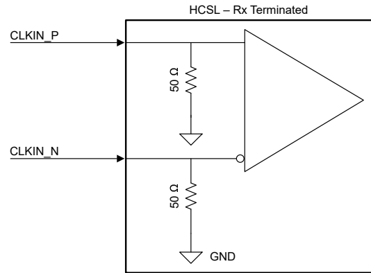
图 8-6. 接收器内部终端
