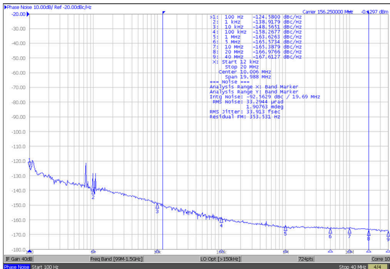
图 6-4. 156.25MHz 时的 LMKDB 输出时钟相位噪声
