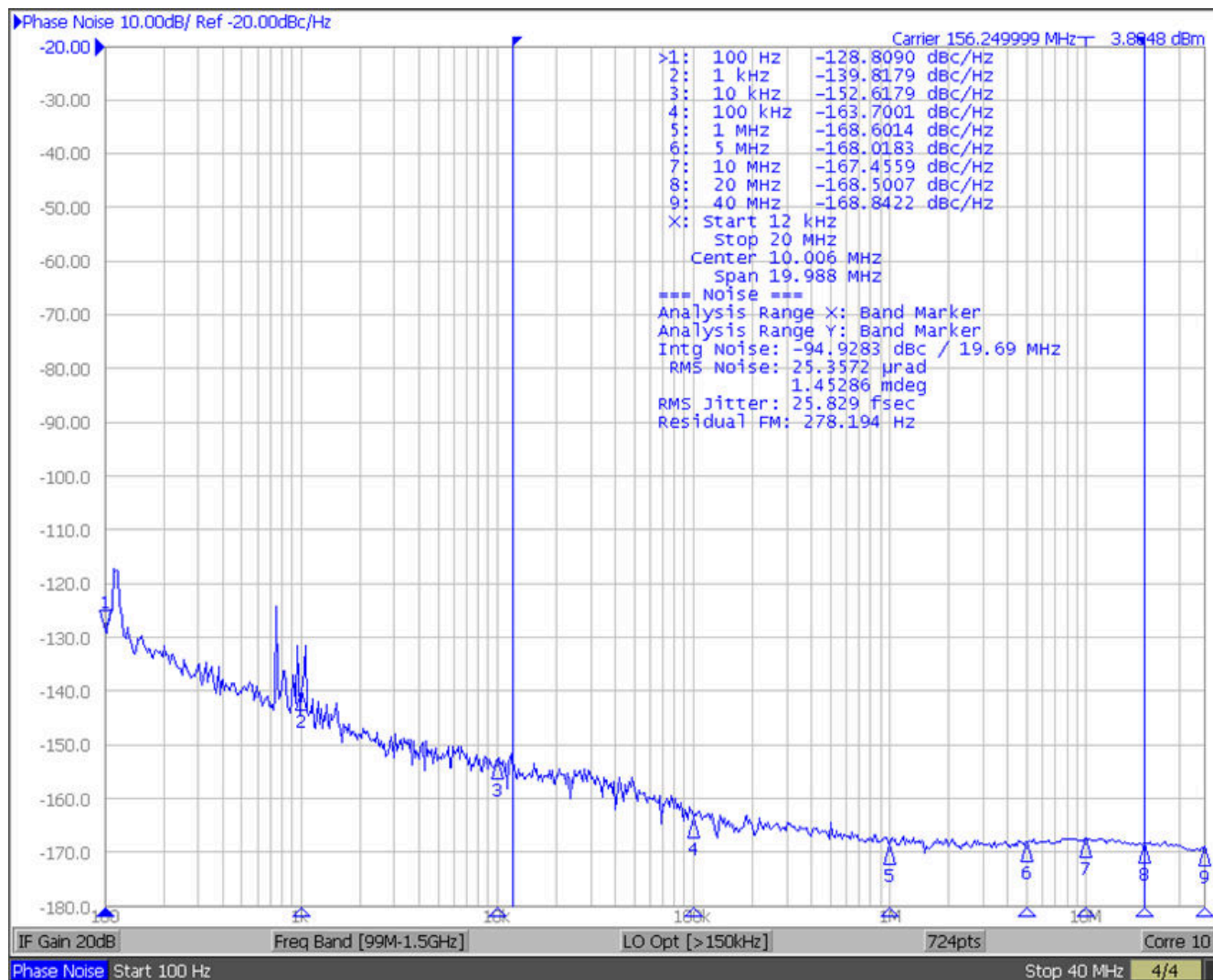
图 10-2. 参考时钟相位噪声
