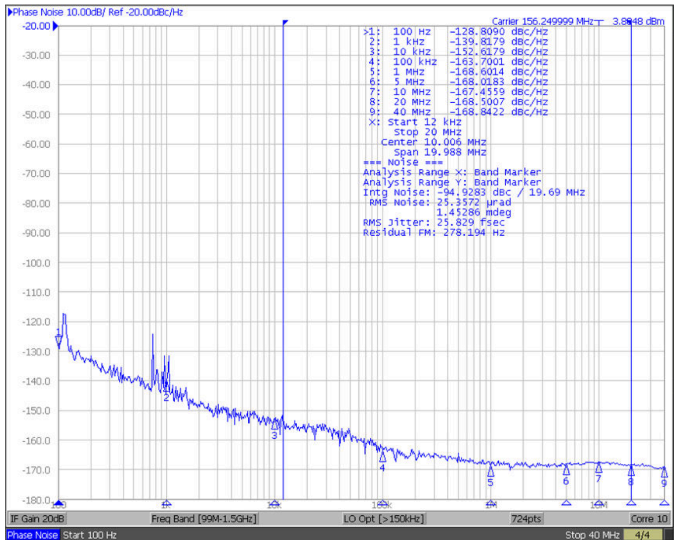
图 6-3. 156.25MHz 时的 LMKDB 输入时钟相位噪声
