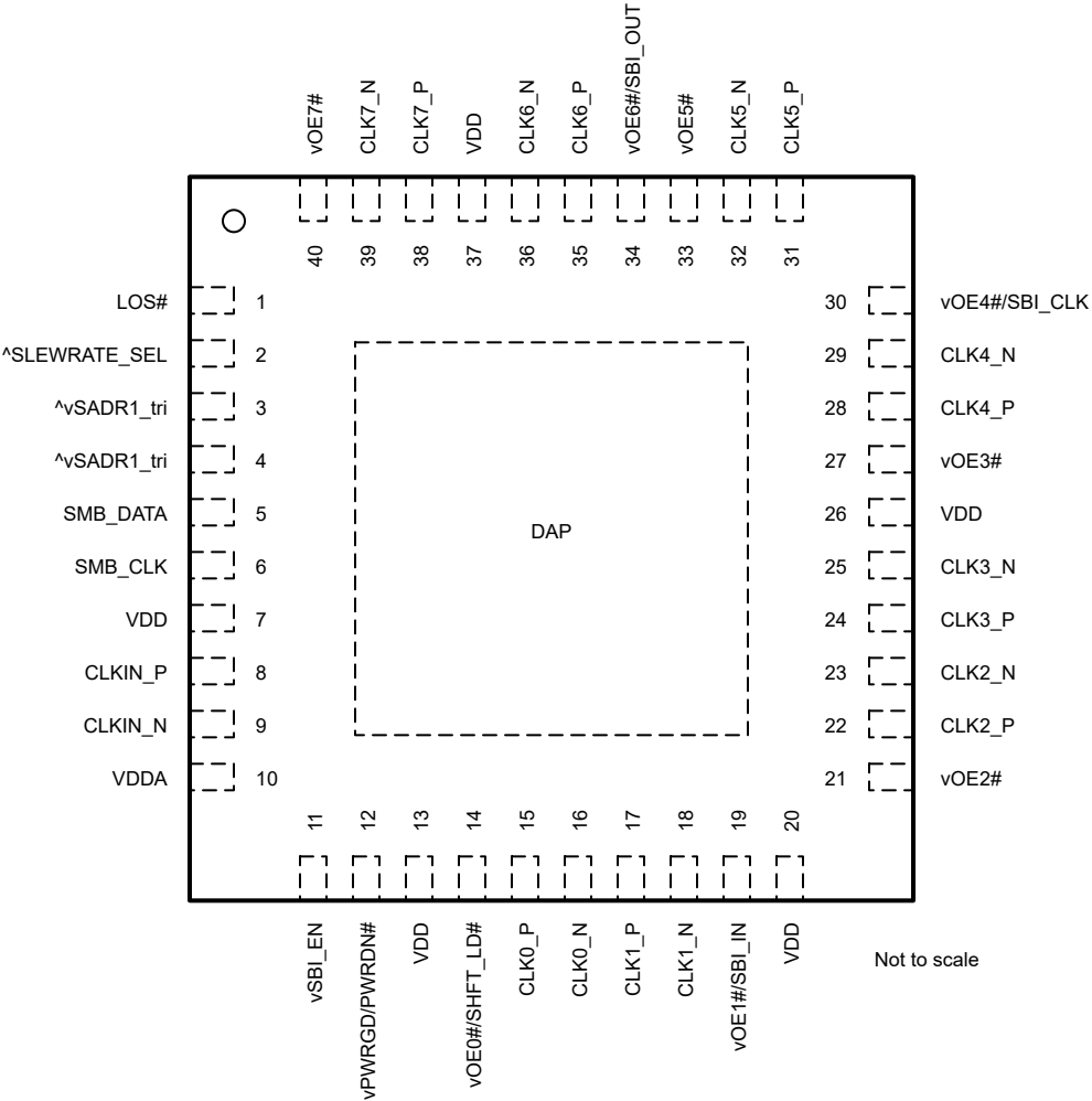
图 5-2. LMKDB1108 RKP 封装，40 引脚 VQFN ( 顶视图 )
