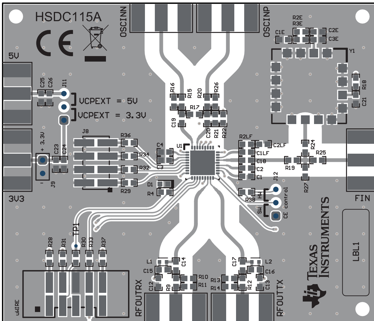
图 10-1. Layout Example
