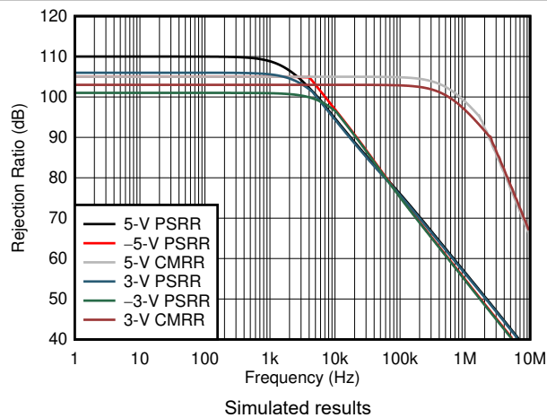
图 7-41. PSRR and CMRR
