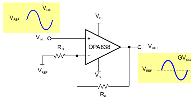
图 8-1. Noninverting Amplifier
