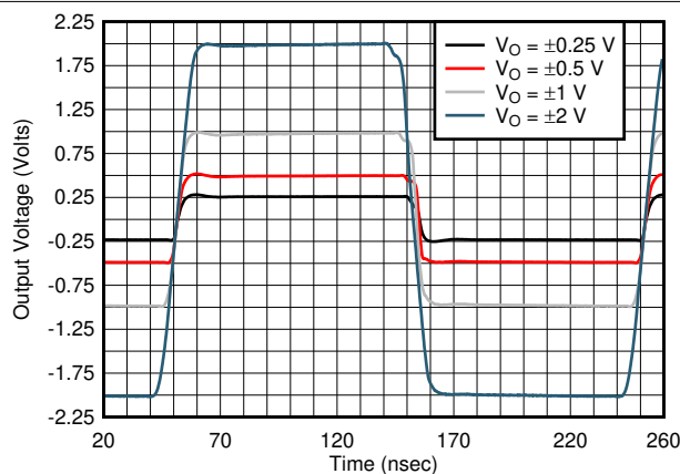
图 7-7. Noninverting Step Response vs V_{OPP}
