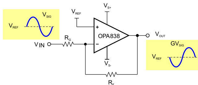
图 8-2. Inverting Amplifier
