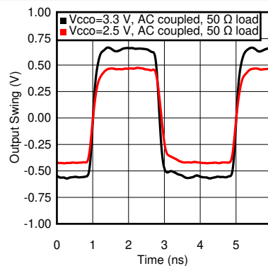
图 6-2. LVCMOS Output Swing at 250 MHz
