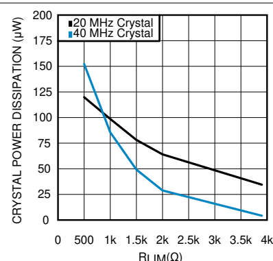
图 6-10. Crystal Power Dissipation vs R LIM
