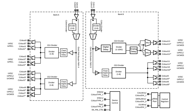
功能方框图
