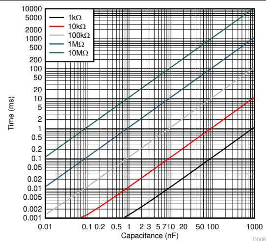
图 6-4. Output Pulse Duration vs Capacitance
