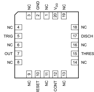
图 4-3. FK Package, 20-Pin LCCC (Top View)
