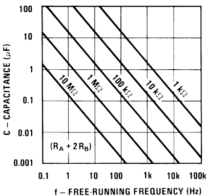
图 7-7. 自由运行频率
