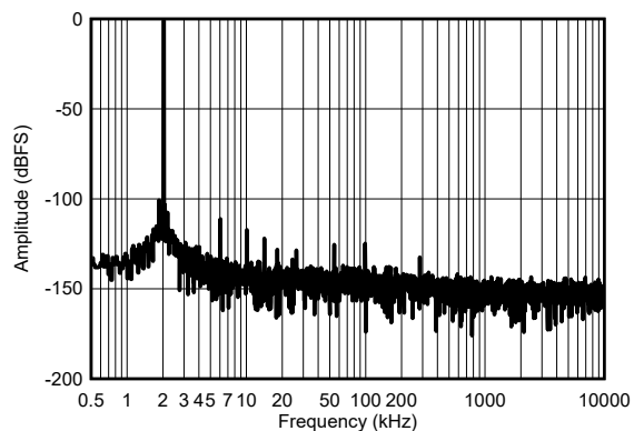
图 5-19. f_{IN} = 2\text{kHz} 时的典型 FFT
