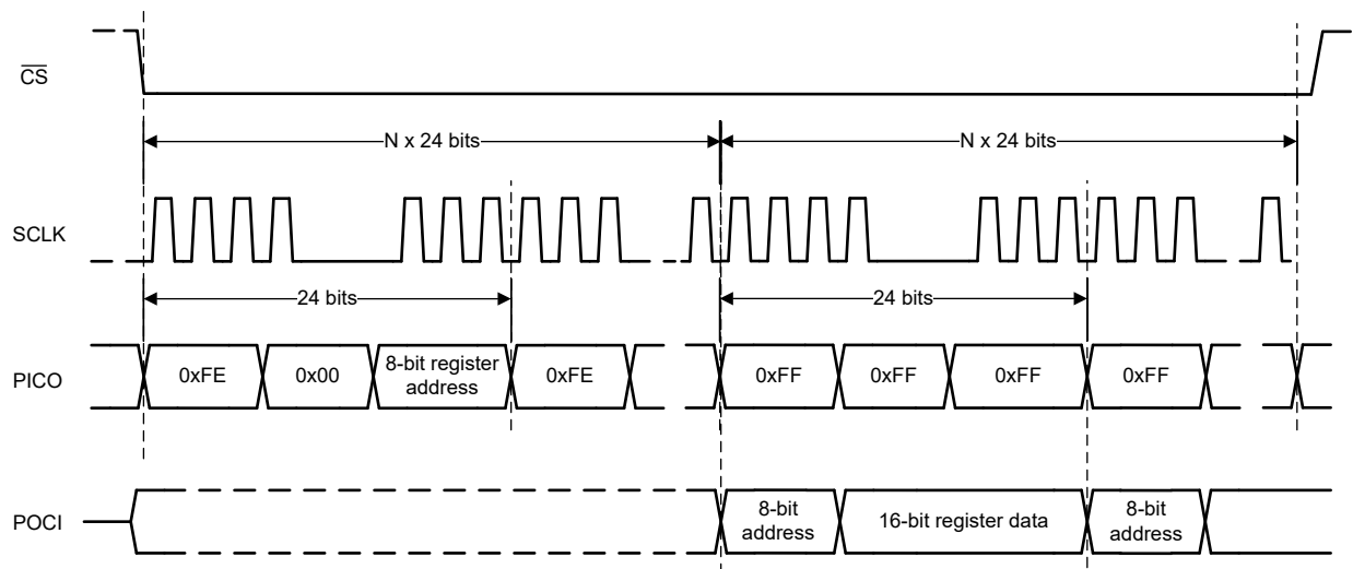
图 6-14. 菊花链配置中的寄存器读取
