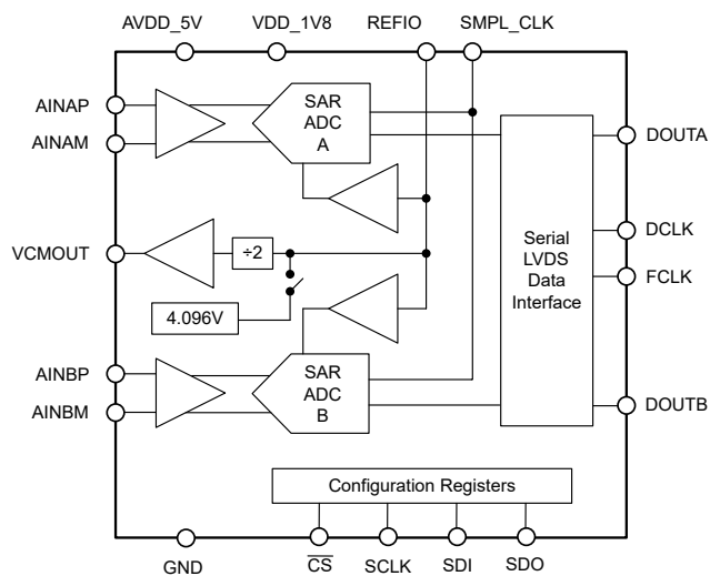
器件方框图
