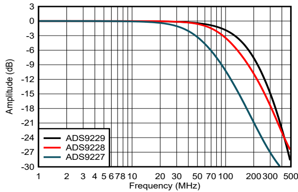
图 5-8. 典型模拟输入带宽
