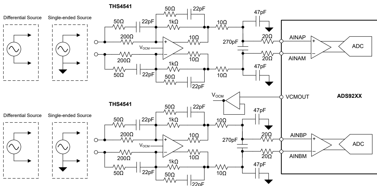
图 8-7. \leq 1\text{MHz} 输入信号带宽的数据采集 (DAQ) 电路
