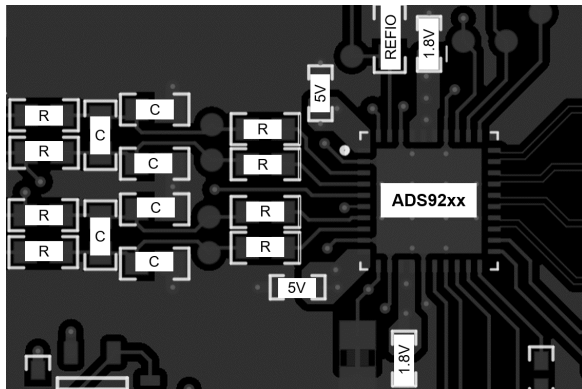
图 8-11. 示例布局
