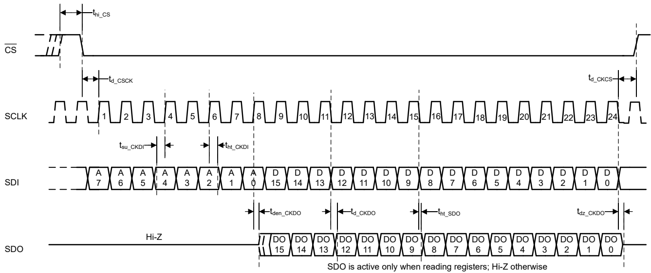
图 5-6. 配置 SPI
