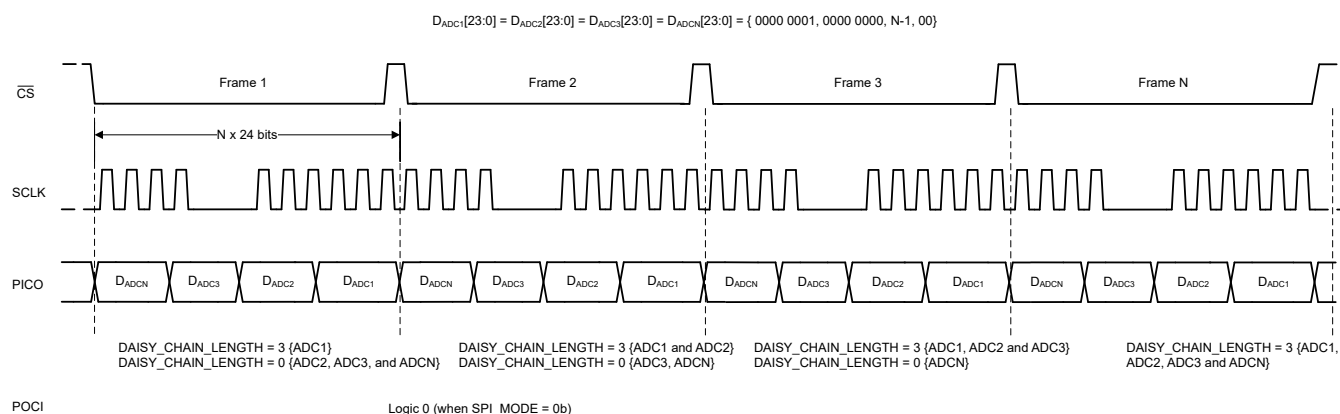
图 6-13. 写入寄存器以配置菊花链长度
