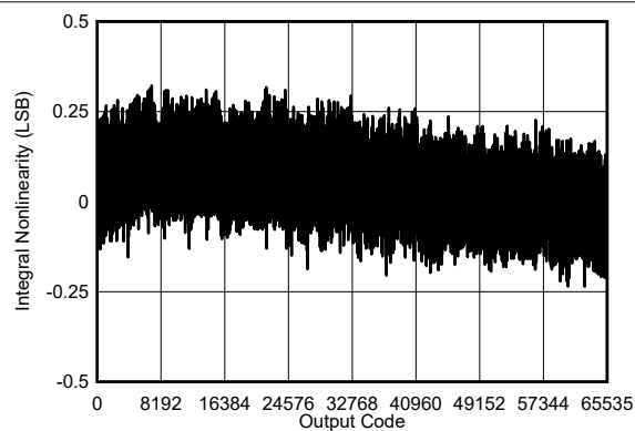
图 8-3. 每通道 5MSPS 时的典型 INL : ADS9227
