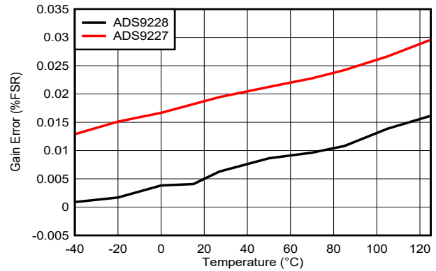
图 5-9. 增益误差与温度间的关系
