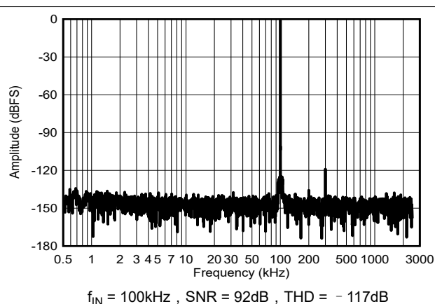
图 8-6. 每通道 5MSPS 时的典型 FFT : ADS9227
