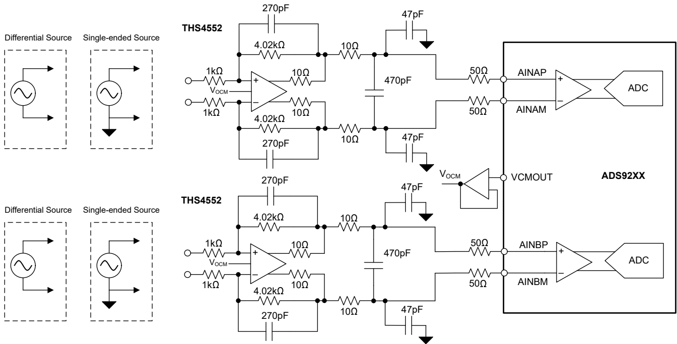
图 8-4. \leq 100\text{kHz} 输入信号带宽的数据采集 (DAQ) 电路
