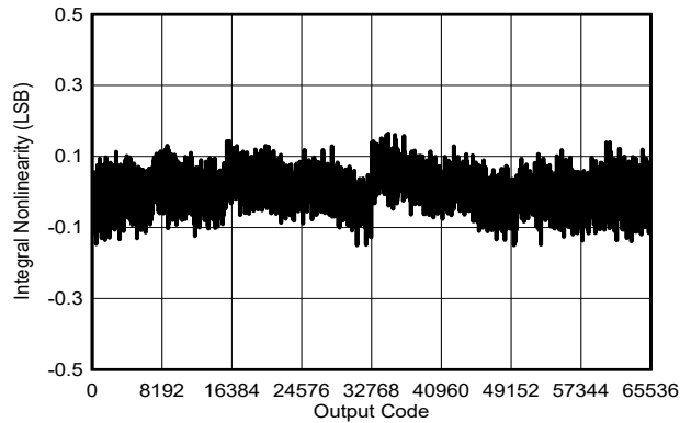
图 5-27. 典型 INL
