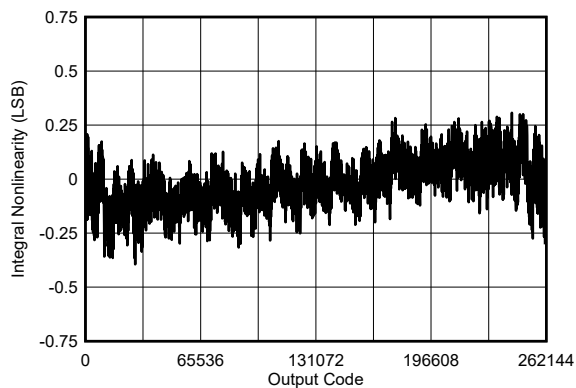
图 5-18. 典型 INL
