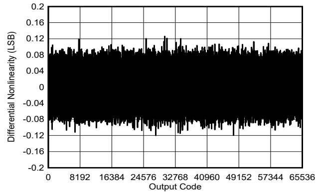
图 5-28. 典型 DNL
