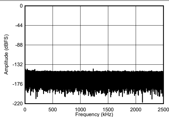
图 8-2. 每通道 5MSPS 时的典型 FFT : ADS9227
