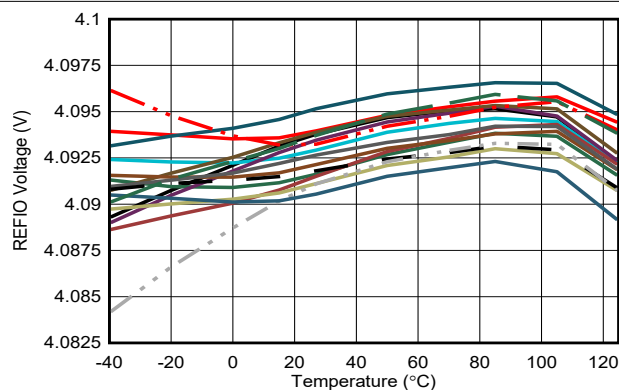
图 5-14. REFIO 电压与温度间的关系
