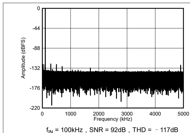
图 8-5. 每通道 10MSPS 时的典型 FFT : ADS9228
