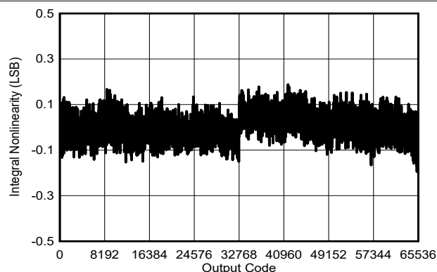
图 5-22. 典型 INL
