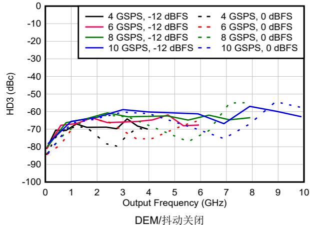
图 6-187. DES2X 模式下 HD3 与频率和采样速率间的关系
