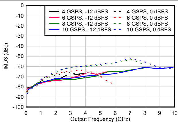
图 6-145. NRZ/RF 模式下 IMD3 与频率和采样速率间的关系
