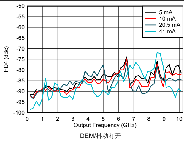
图 6-189. NRZ/RF 模式下 HD4 与频率和输出电流间的关系
