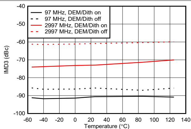
图 6-149. DES2XL 模式下 IMD3 与温度间的关系
