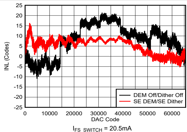
图 6-13. INL 与 DAC 代码间的关系：20.5mA
