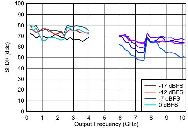
图 6-121. DES2X 模式下 SFDR 与频率和数字振幅间的关系
