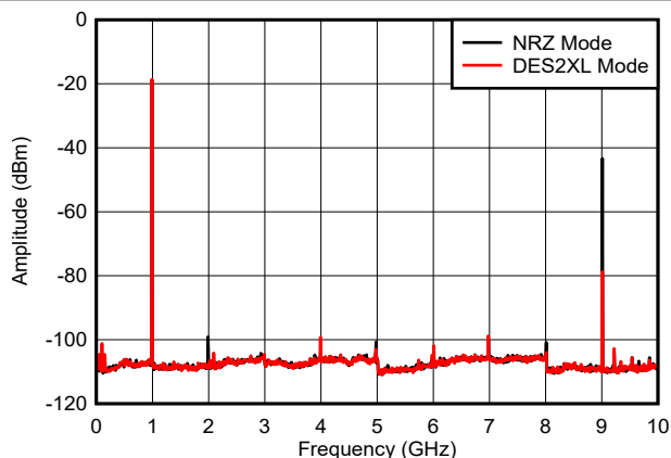
图 6-22. f_{\text{OUT}} = 997\text{MHz} ， 0\text{dBFS}
