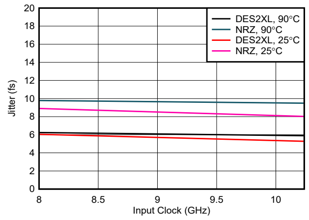
从 100Hz 集成到 30MHz，DEM/抖动关闭
