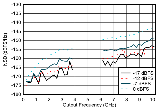
图 6-70. NSD 与输出频率和数字振幅间的关系
