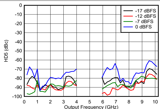
图 6-201. DES2X 模式下 HD5 与频率和数字振幅间的关系
