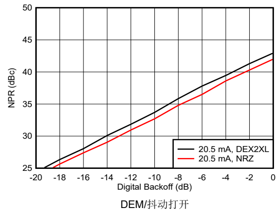
图 6-213. 噪声功率比与数字退避间的关系：第二奈奎斯特区域
