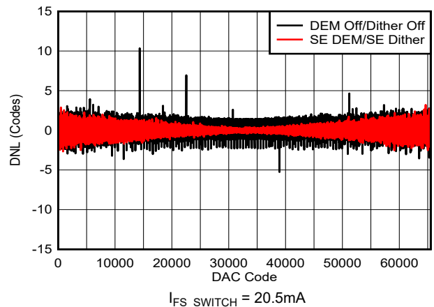
图 6-11. DNL 与 DAC 代码间的关系：20.5mA
