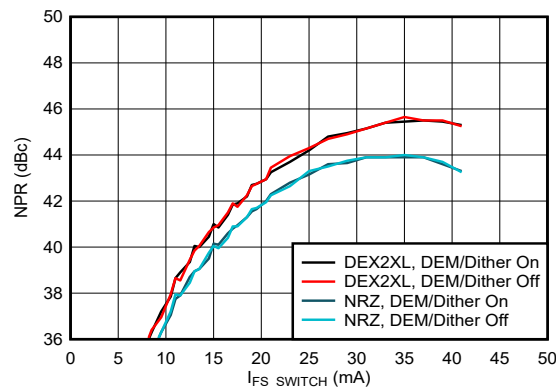
图 6-215. 电源抑制比与输出电流间的关系：第二奈奎斯特区域
