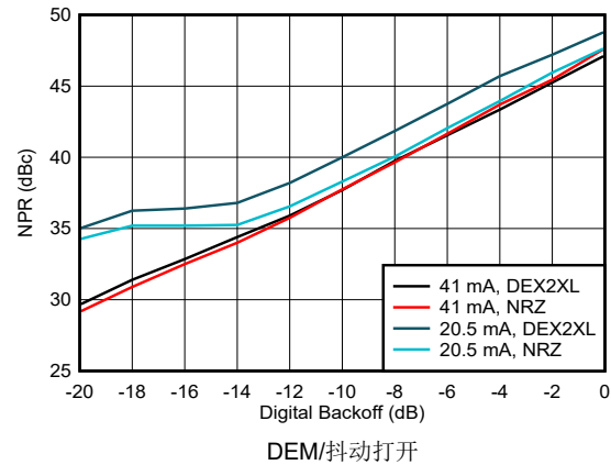
图 6-211. 噪声功率比与数字退避间的关系：第一奈奎斯特区域
