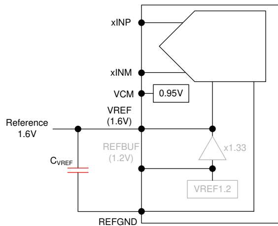
图 7-15. External 1.6V reference
