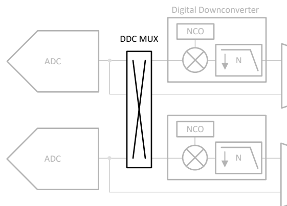
图 7-18. DDC MUX
