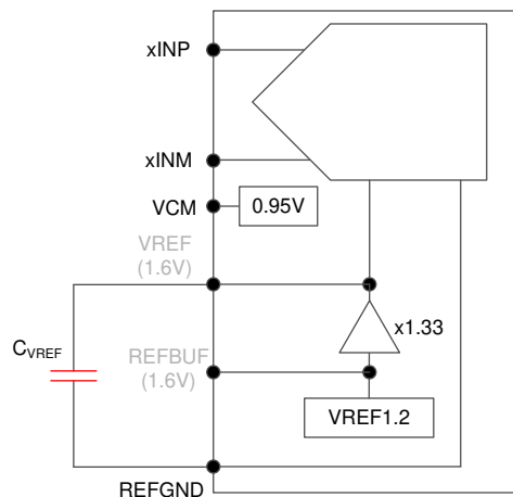
图 7-14. Internal reference
