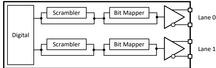
图 7-37. Output scrambling per lane
