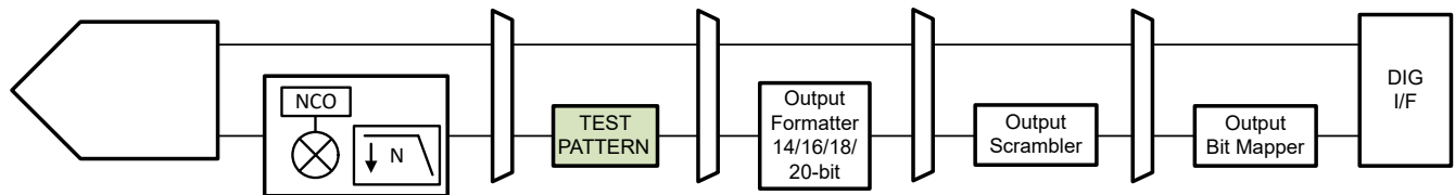
图 7-44. Test Pattern Generator
