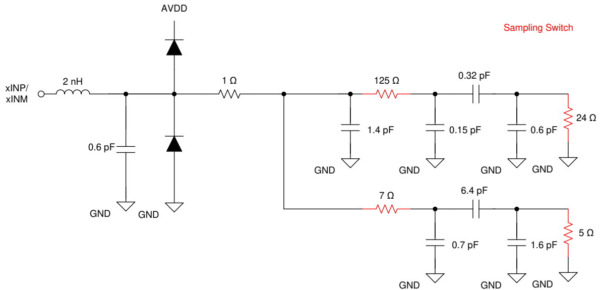
图 7-1. Equivalent input network
