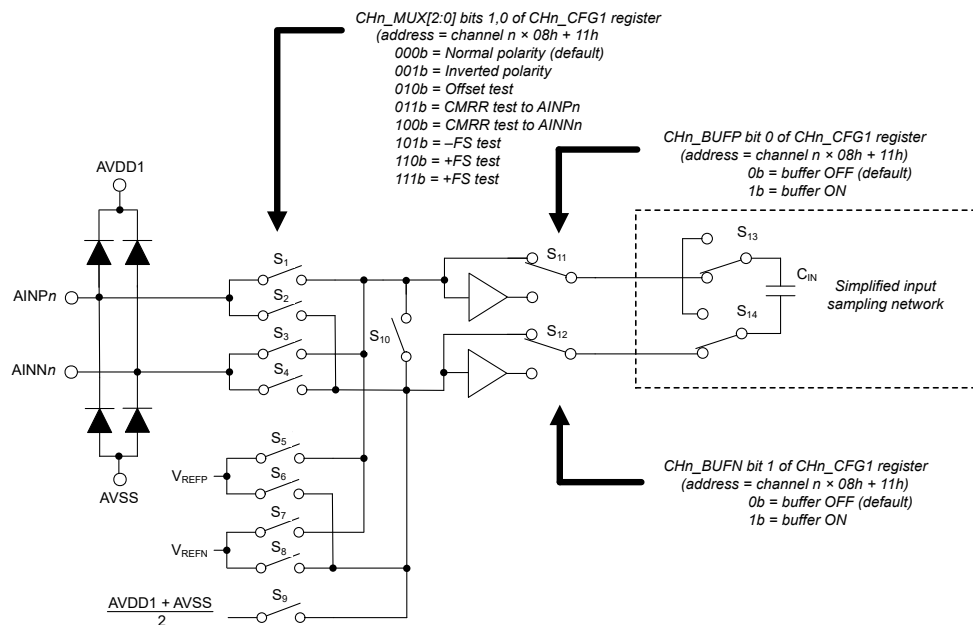
图 7-3. Analog Input Circuit
