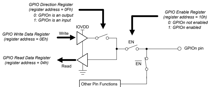
图 7-9. GPIO Block Diagram
