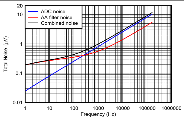
图 9-5. Total Noise
