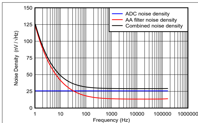
图 9-4. Noise Density
