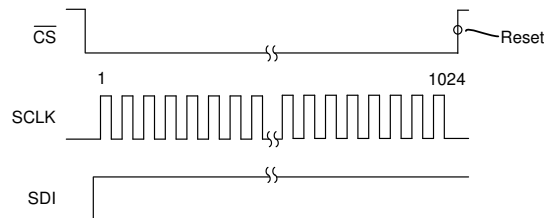
图 7-29. SPI Reset Pattern
