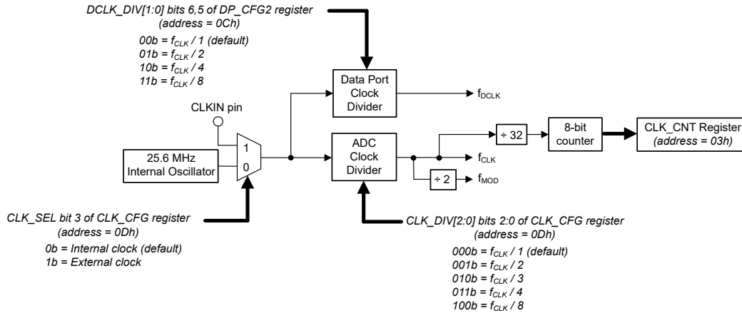
图 7-6. Clock Block Diagram
