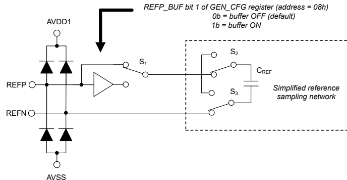
图 7-5. Reference Input Circuit
