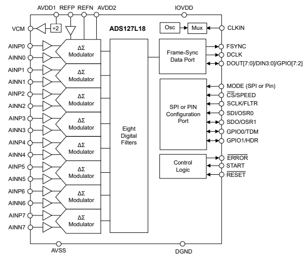
功能方框图
