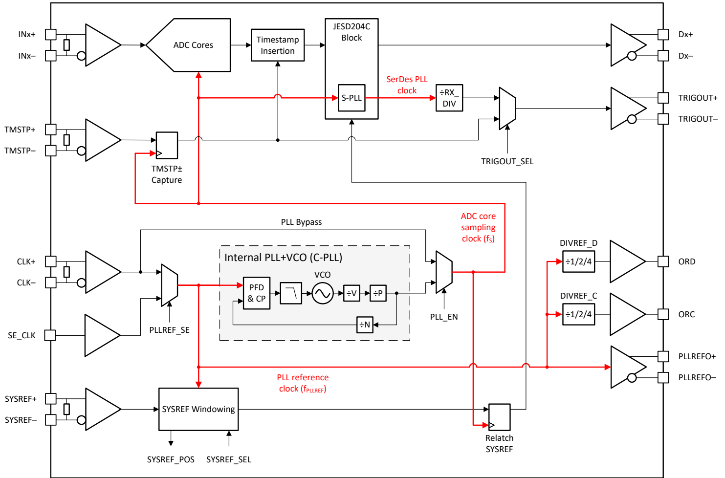
图 6-3. Clocking Subsystem
