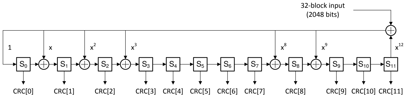
图 6-7. CRC-12 Parity Bit Generator
