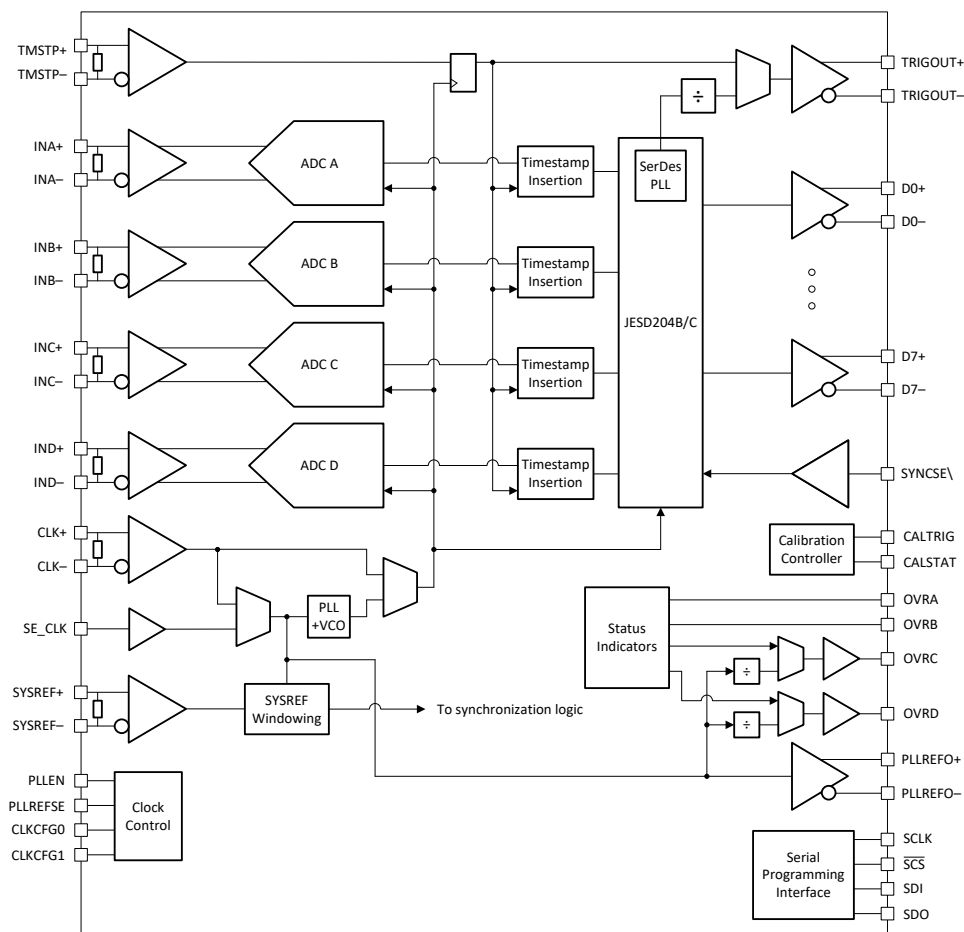
四通道器件方框图
