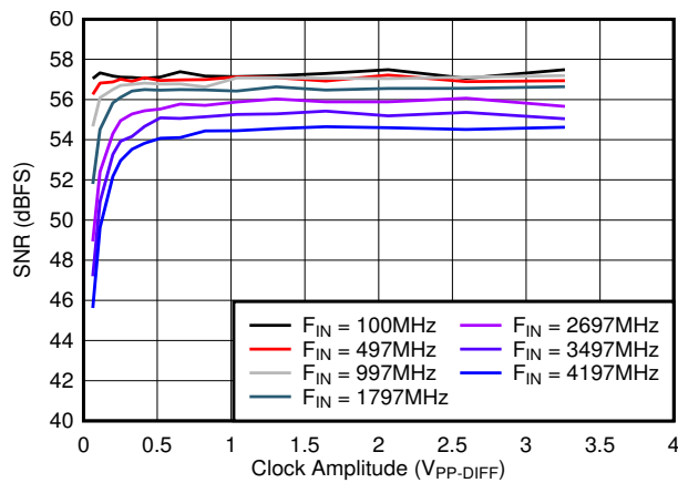
图 5-37. SNR vs A_{CLK}
