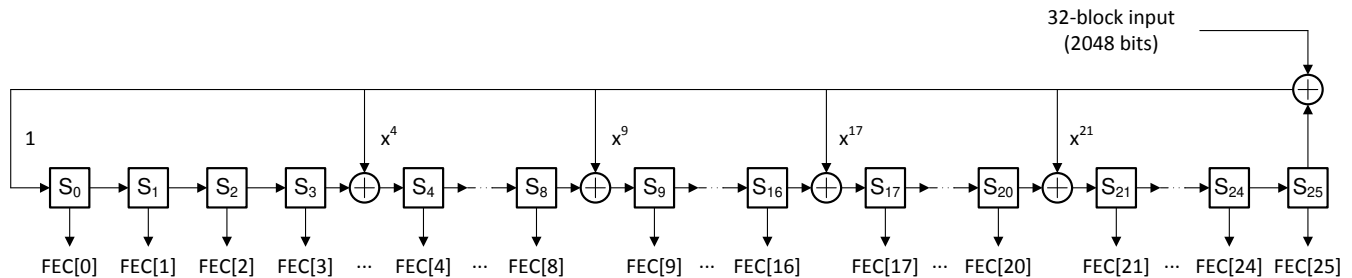
图 6-8. FEC Parity Bit Generator
