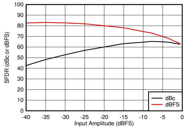
图 5-34. SFDR vs A_{IN}
