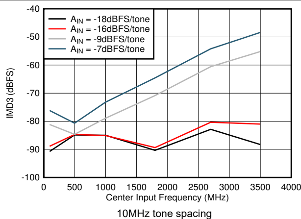
图 7-75. IMD3 vs F_{IN}
