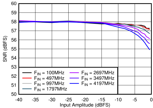
图 7-33. SNR vs A_{IN}
