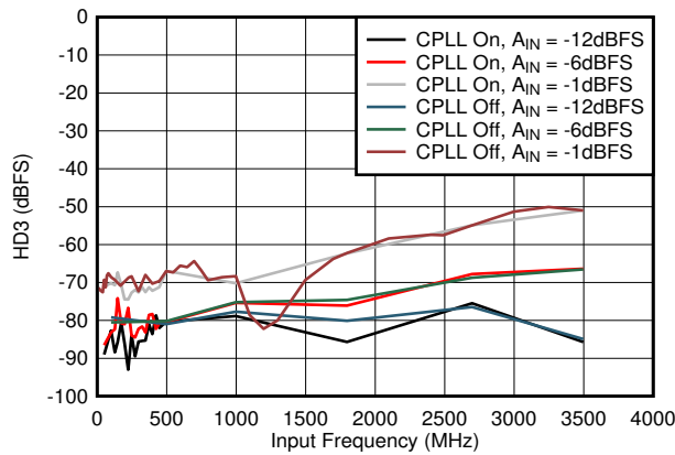
图 7-53. HD3 vs A_{IN} and C-PLL
