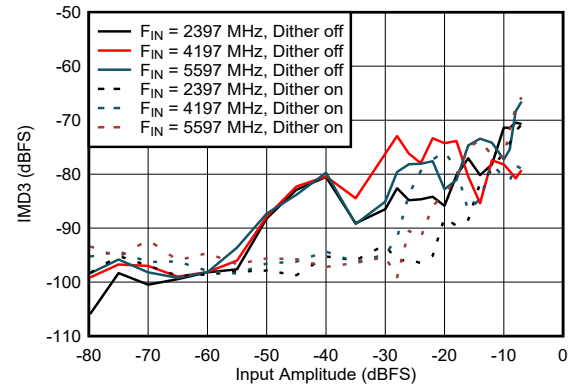
图 5-24. DES Mode: IMD3 vs Input Amplitude
