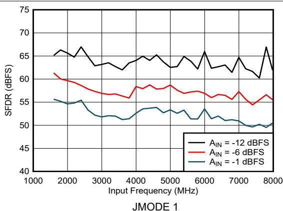
图 5-9. DES Mode: SFDR vs Input Frequency
