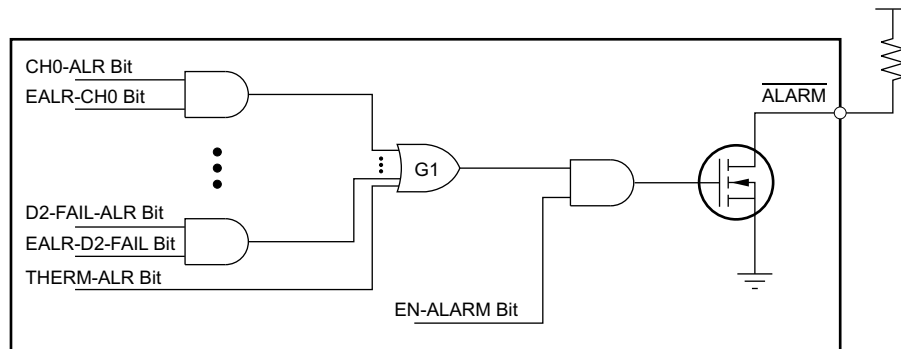
图 7-15. \overline{\text{ALARM}} Pin
