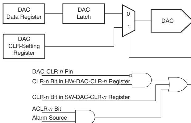
图 7-11. Clearing DAC- n
