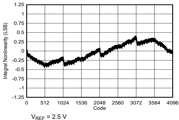
图 6-7. Integral Linearity Error vs Code
