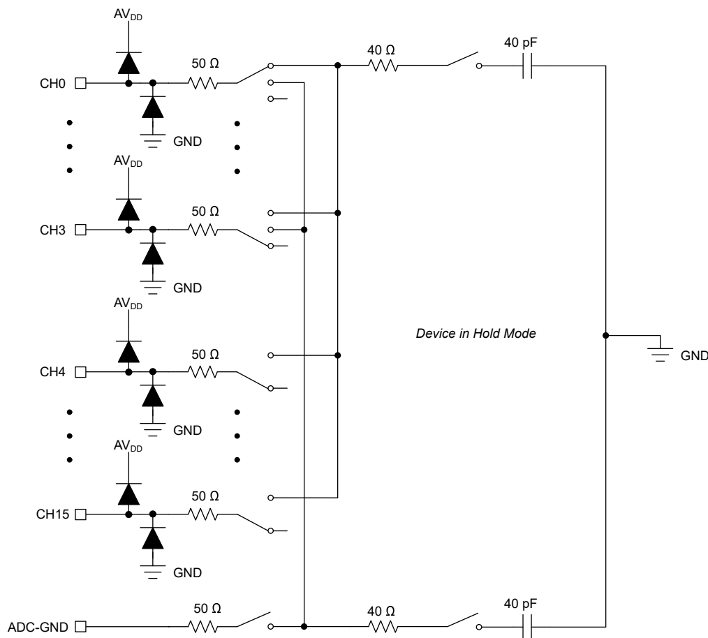
图 7-1. Equivalent Input Circuit
