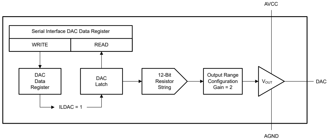
图 7-9. DAC Block Diagram
