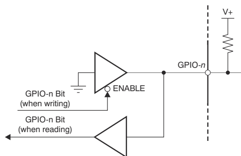
图 7-17. GPIO Pins
