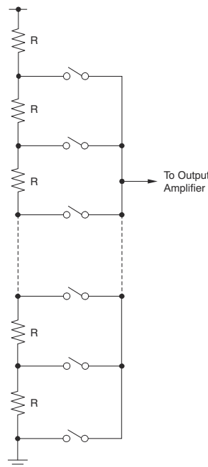
图 7-10. Resistor String
