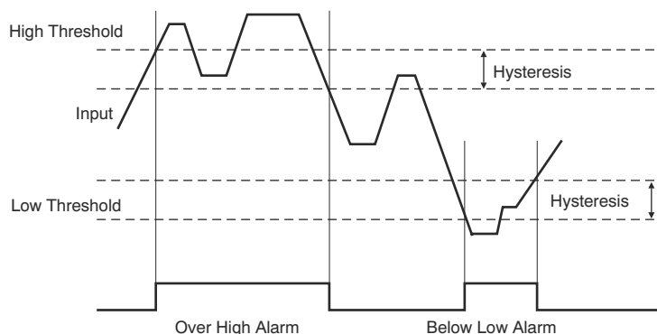
图 7-16. Hysteresis
