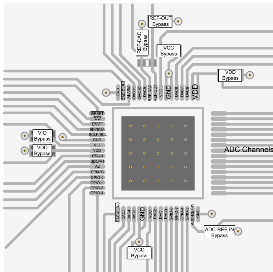
图 8-6. AFE11612-SEP Layout Example
