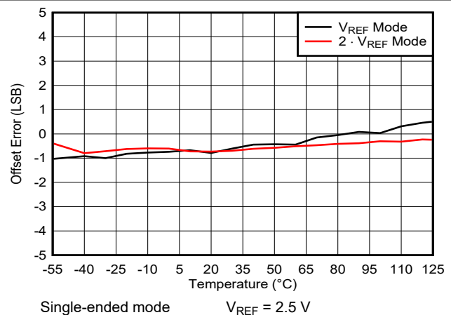
图 6-37. Offset vs Temperature
